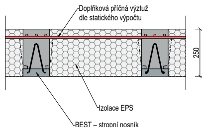
PŘÍČNÝ ŘEZ
