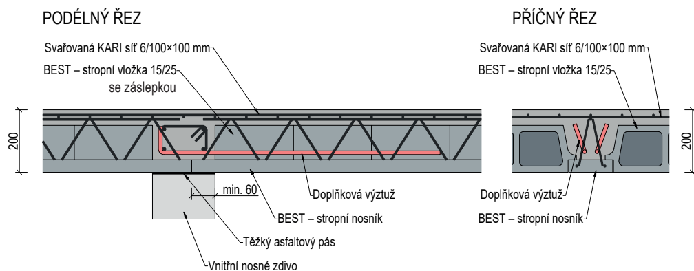
DOPLŇKOVÁ VÝZTUŽ
