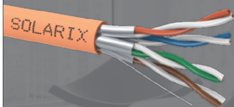
Instalační kabel Solarix CAT6A STP ISOHR B2 ca s1 d1 a1
