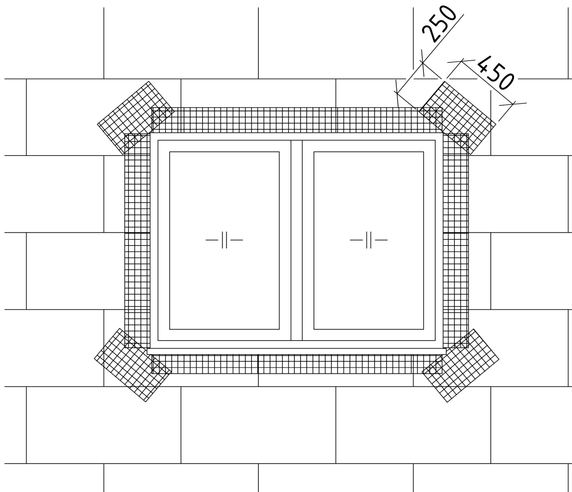
Obrázek 18 - zesílení výztužné vrstvy v okolí okenního otvoru
