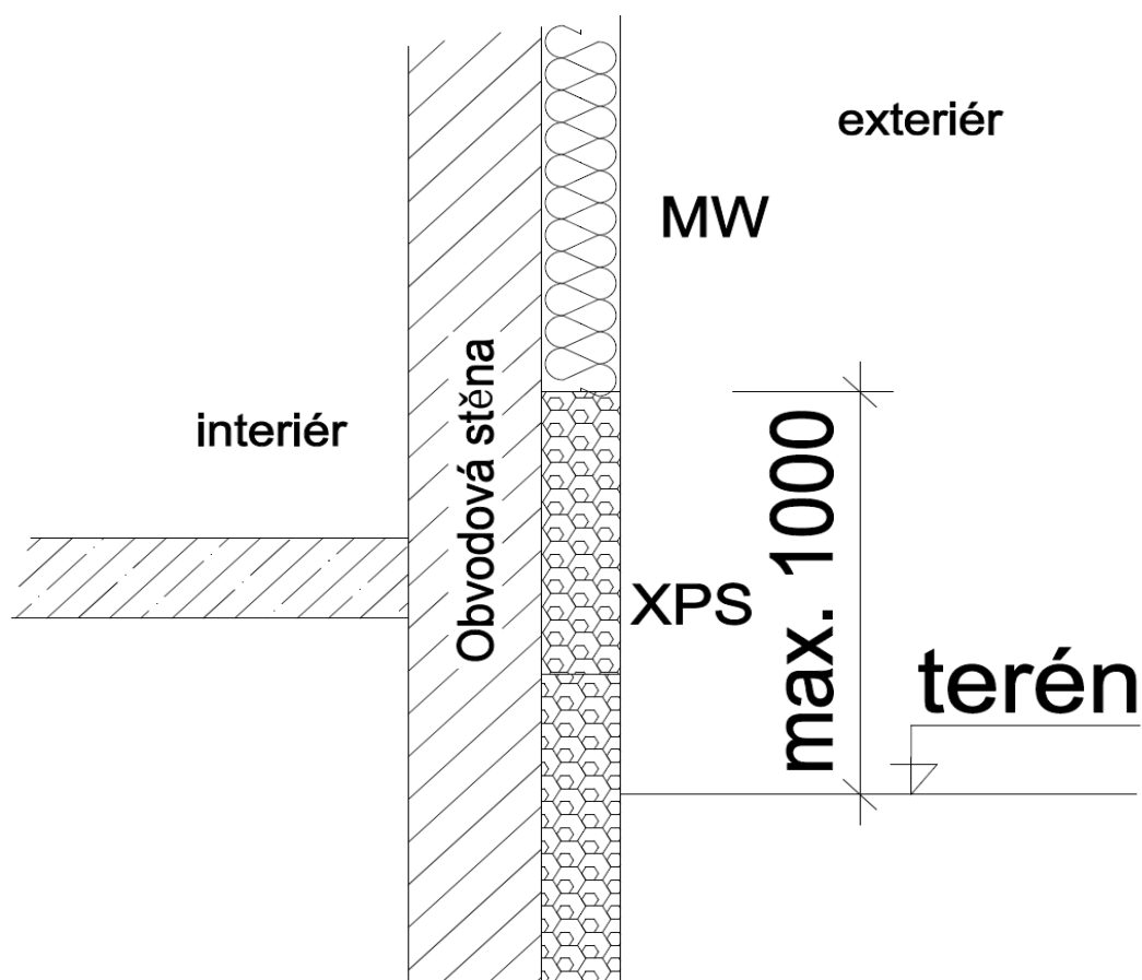
Obrázek 7 – Detail zateplení soklu objektu se založením ETICS pod terénem dle bodu a1 s požární výškou h > 22,5 \text{ m} dle požadavků ČSN 73 0810
