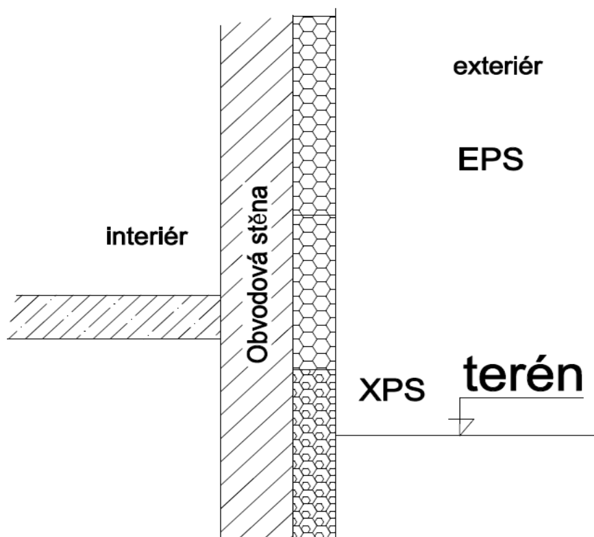
Obrázek 5 – Detail zateplení soklu objektu se založením ETICS pod terénem dle bodu a1 s požární výškou 12,0 < h \leq 22,5 m dle požadavků ČSN 70810
