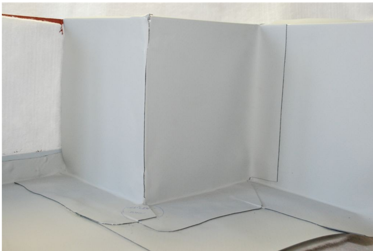
Obrázek 13.: Postup opracování hydroizolace na rohu
