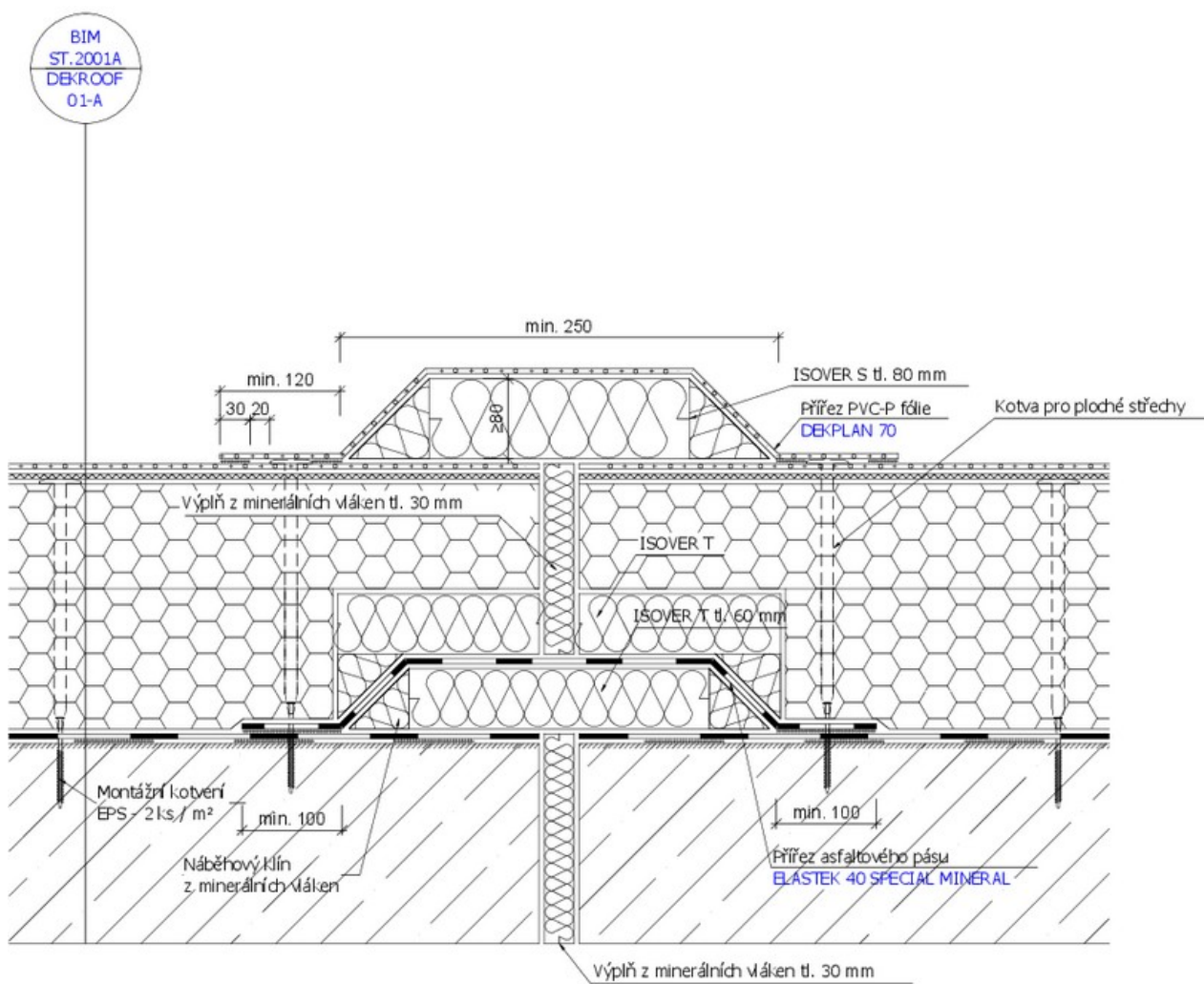
Detail 7.: Objektová dilatační spára svislý/vodorovný posun 20-30 mm
