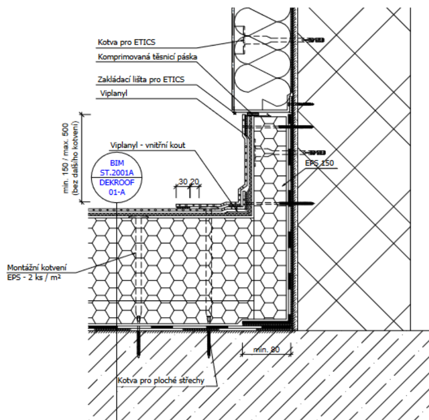
Detail 3.:Detail napojení vodorovné a svislé plochy, detail ukončení fólie na svislé ploše
