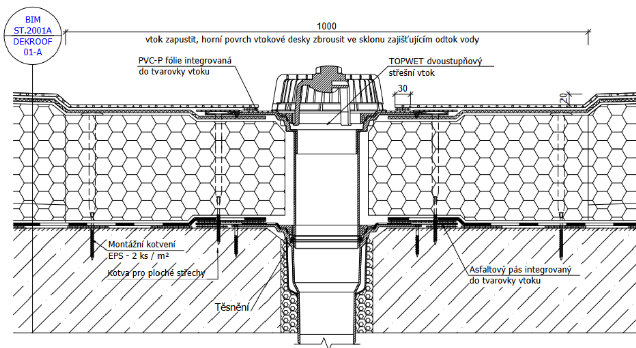
Detail 9.: Opracování střešního vtoku (manžetu vtoku je možné napojit na hydroizolaci z plochy jak ze spodní tak i z horní strany)
