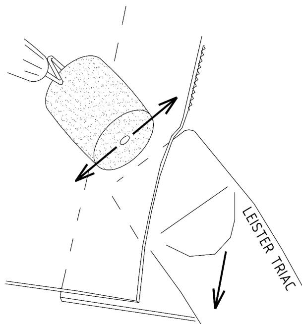
Obrázek 4.: Práce s horkovzdušným přístrojem a válečkem
