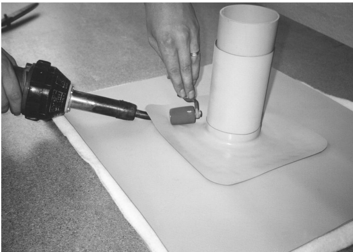
Obrázek 22.: Opracování prostupu - celoplošné navaření manžety k fólii v ploše
