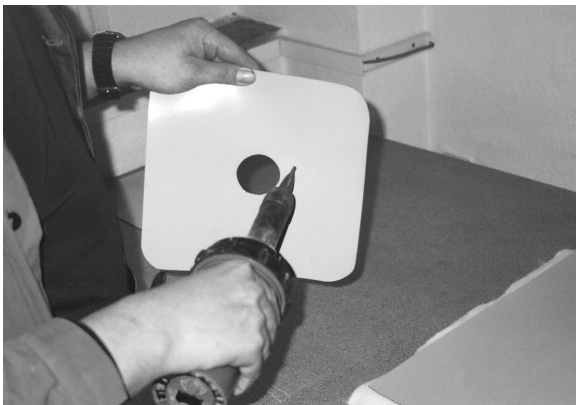
Obrázek 19.: Opracování prostupu - nahřívání manžety pouze z rubové strany
