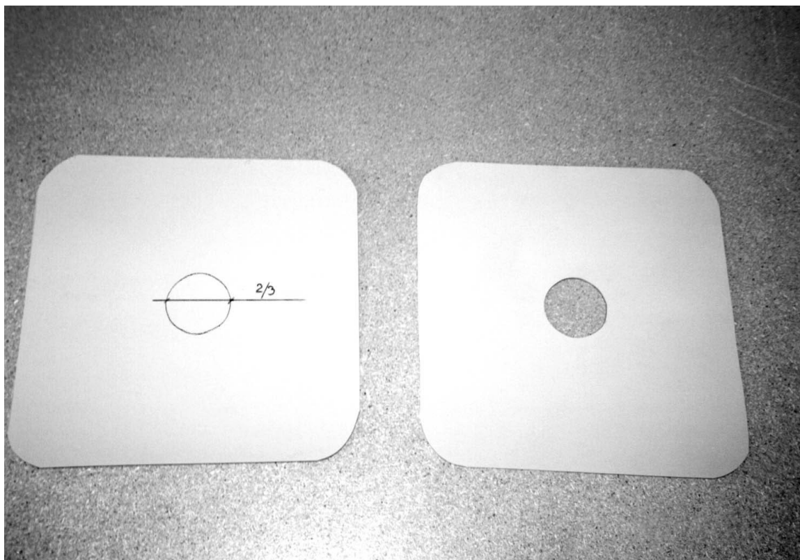
Obrázek 18.: Opracování prostupu - příprava manžety
