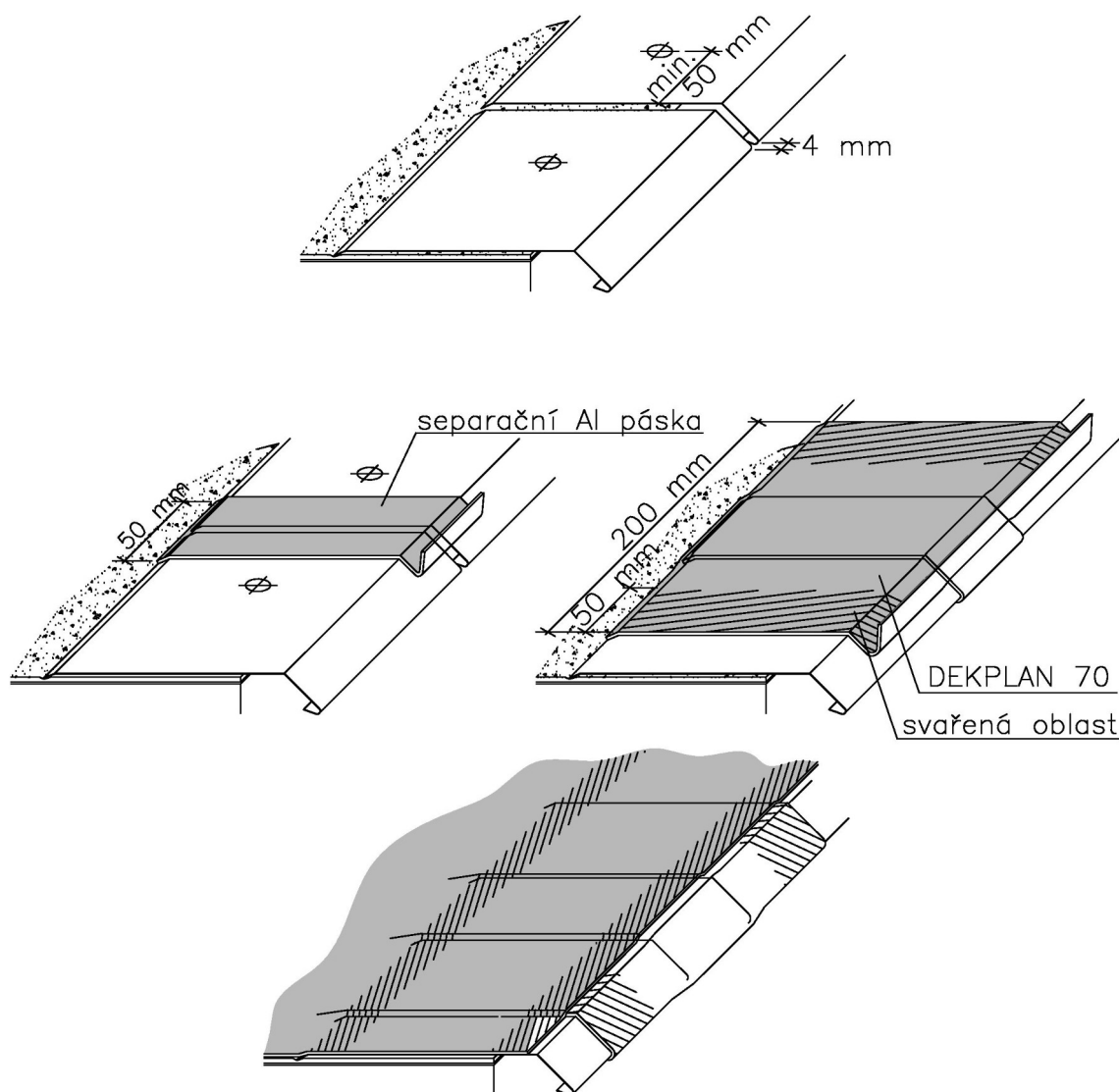
Obrázek 6.: Postup ukončení hydroizolace na profilu ze spojovacího plechu
