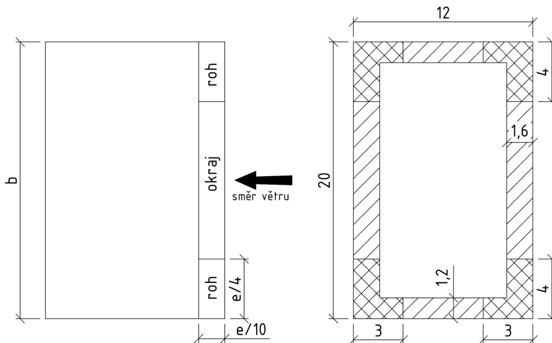
Obrázek 2.: Příklad rozdělení ploché střechy dle zatížení větrem
