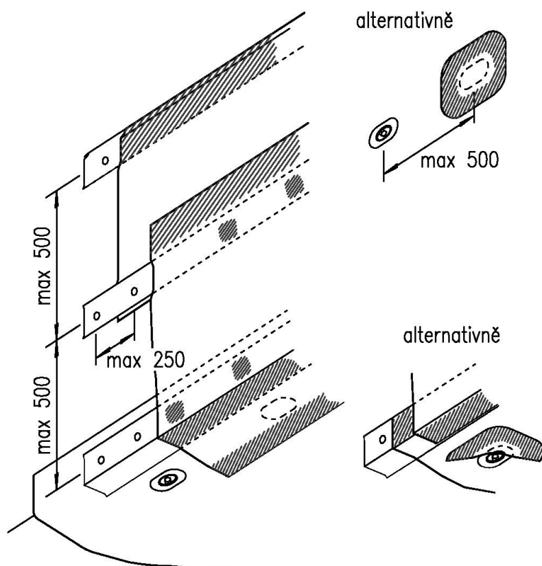
Obrázek 7.: Vytažení hydroizolace na svislou konstrukci
