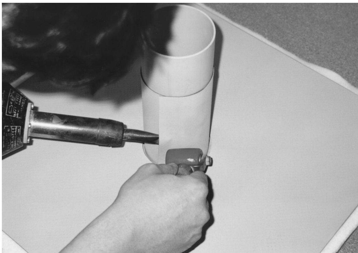
Obrázek 17.: Opracování prostupu - navaření pásku na kruhový prostup
