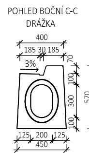
BEST TROUBA SE ŠTĚRBINOVÝM ŽLABEM, NÁBĚHOVÁ 0-7, OBRUBNÍK 7 cm, (PROFIL LEVÝ)
