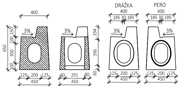
ŘEZ A-A ŘEZ B-B POHLED BOČNÍ D-D DŘÁŽKA POHLED BOČNÍ C-C PERO
