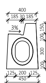
POHLED BOČNÍ D-D DRÁŽKA
