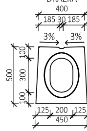
BEST ZÁSLEPKA TROUBY SE ŠTĚRBINOVÝM ŽLABEM ZAKONČENÁ PEREM
