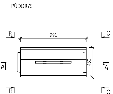
BEST TROUBA SE ŠTĚRBINOVÝM ŽLABEM, NÁBĚHOVÁ 0-7, OBRUBNÍK 7 cm, (PROFIL LEVÝ)
