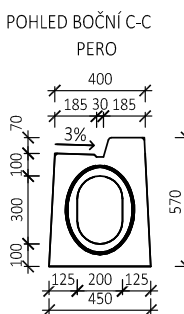
BEST TROUBA SE ŠTĚRBINOVÝM ŽLABEM, NÁBĚHOVÁ 7-0, OBRUBNÍK 7 cm, (PROFIL PRAVÝ)
