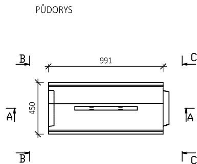
BEST TROUBA SE ŠTĚRBINOVÝM ŽLABEM, NÁBĚHOVÁ 7-0, OBRUBNÍK 7 cm, (PROFIL PRAVÝ)
