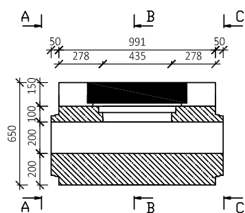
POHLED BOČNÍ A-A PERO
