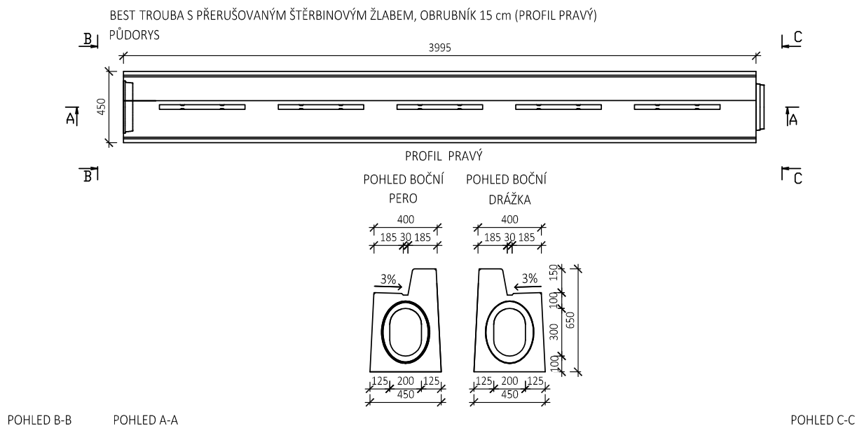
BEST TROUBA S PŘERUŠOVANÝM ŠTĚRBINOVÝM ŽLABEM, ROVNÁ, OBRUBNÍK 15 cm (PROFIL PRAVÝ)
