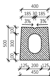
BEST ZÁSLEPKA TROUBY SE ŠTĚRBINOVÝM ŽLABEM ZAKONČENÁ DŘÁŽKOU
