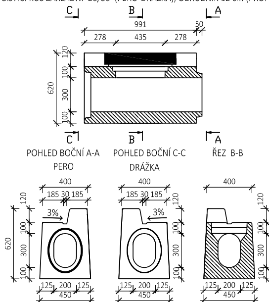
BEST VPUŠŤOVÝ KUS 20/30 (PERO-DŘÁŽKA), OBRUBNÍK 12 cm (PROFIL PRAVÝ)
