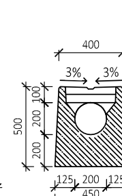
ŘEZ B-B
