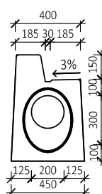
POHLED BOČNÍ C-C PERO
