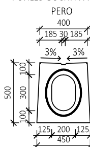
POHLED BOČNÍ A-A
