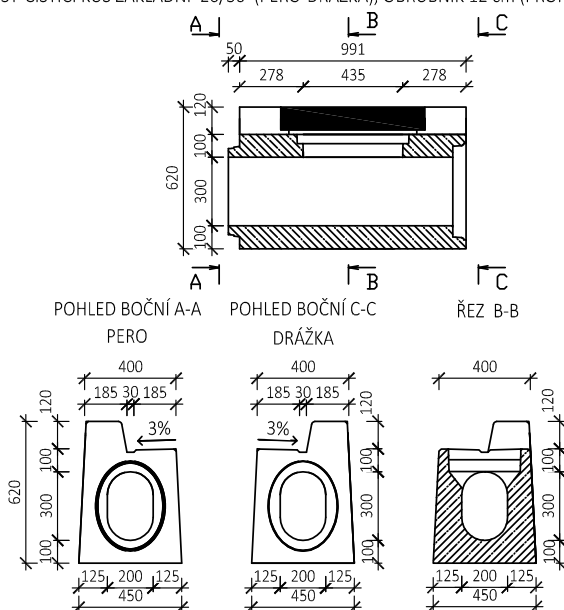
BEST VPUŠŤOVÝ KUS 20/30 (PERO-DŘÁŽKA), OBRUBNÍK 12 cm (PROFIL LEVÝ)
