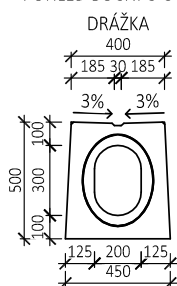
POHLED BOČNÍ C-C
