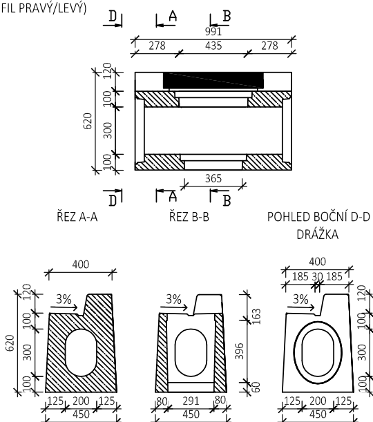
BEST VPUŠŤOVÝ KUS (DŘÁŽKA-DŘÁŽKA), OBRUBNÍK 12 cm (PROFIL PRAVÝ/LEVÝ)
