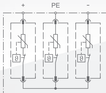
SCHÉMA ZAPOJENÍ
