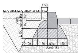
Osadenie cestných obrubníkov
