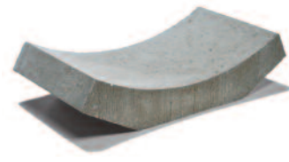
Priekopová tvárnica formát: 59 x 33 x 15,8 cm farba: sivá prehĺbenie: 7,8 cm
