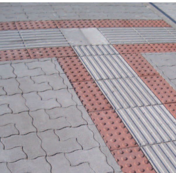
Dlažba pre nevidiacich formát: 40 x 40 x 8 cm, s drážkami farby: sivá, červená
