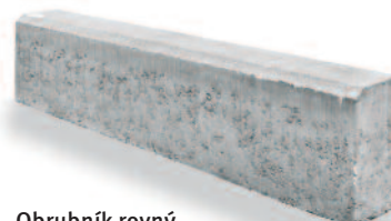
Obrubník rovný formát: 100 x 20 x 10 cm, 100 x 25 x 15 cm, 100 x 25 x 8 cm
