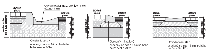
Osadenie žľabov a nájazdových obrubníkov
