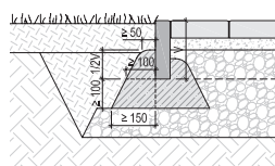
Osadenie parkových obrubníkov
