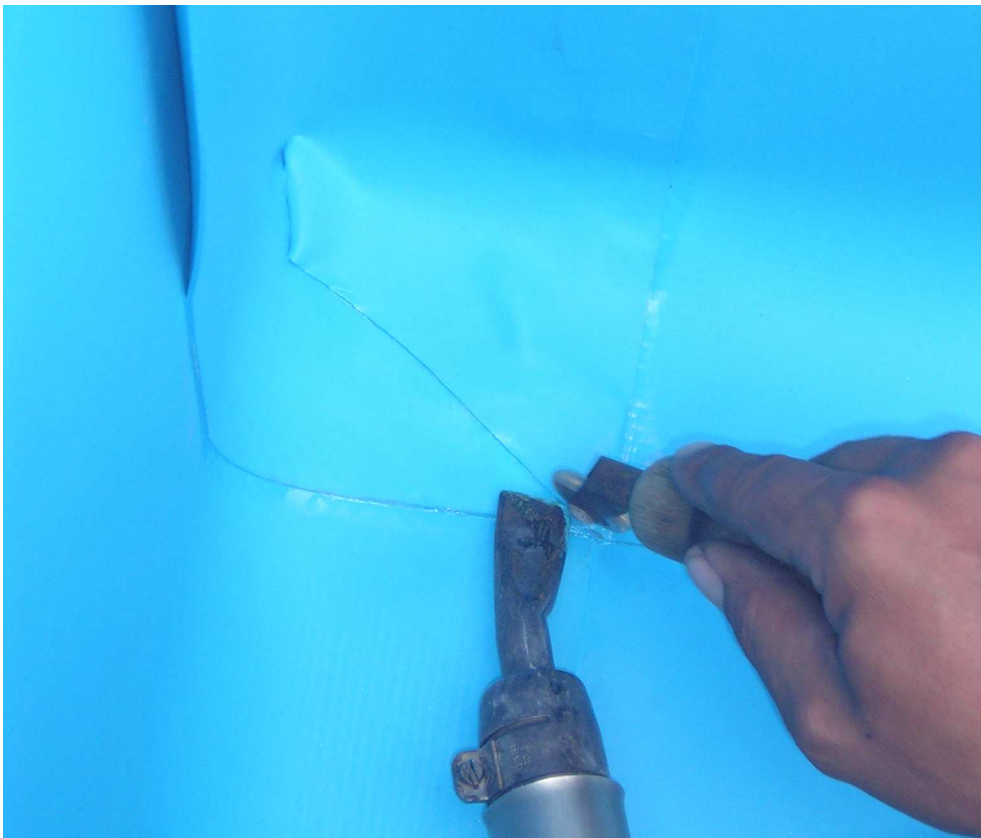
Foto 6. Správne zhotovený kút, spôsob I.
