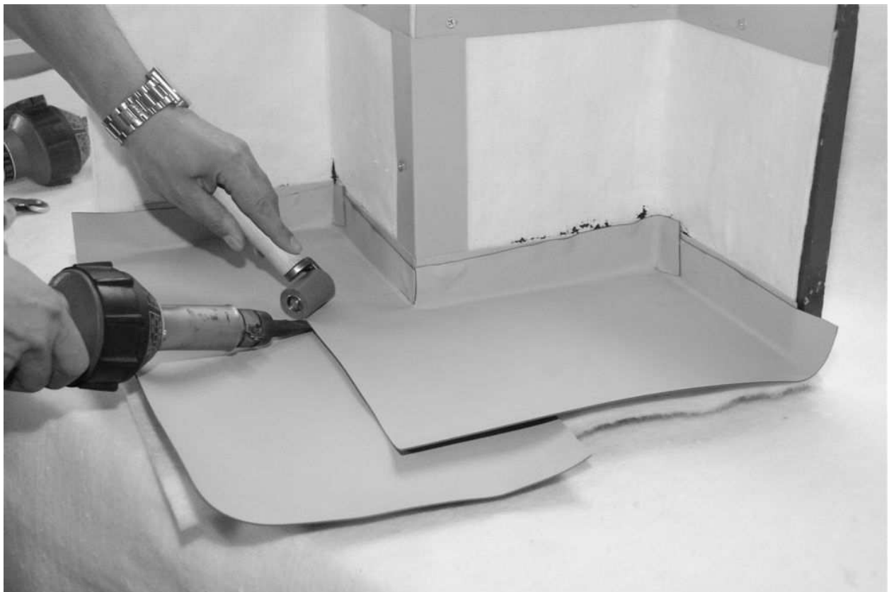
Obrázek 10.: Postup opracování hydroizolace na rohu
