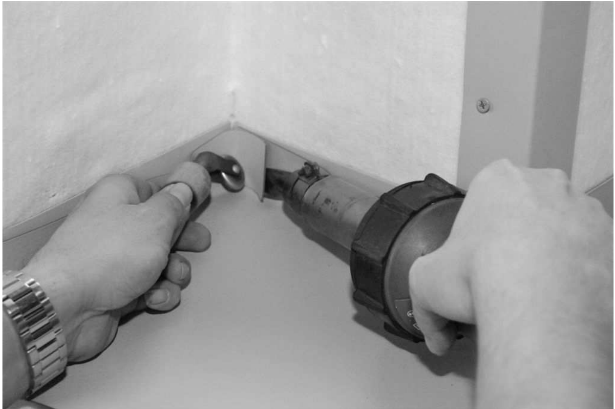
Obrázek 9.: Postup opracování hydroizolace v koutu
