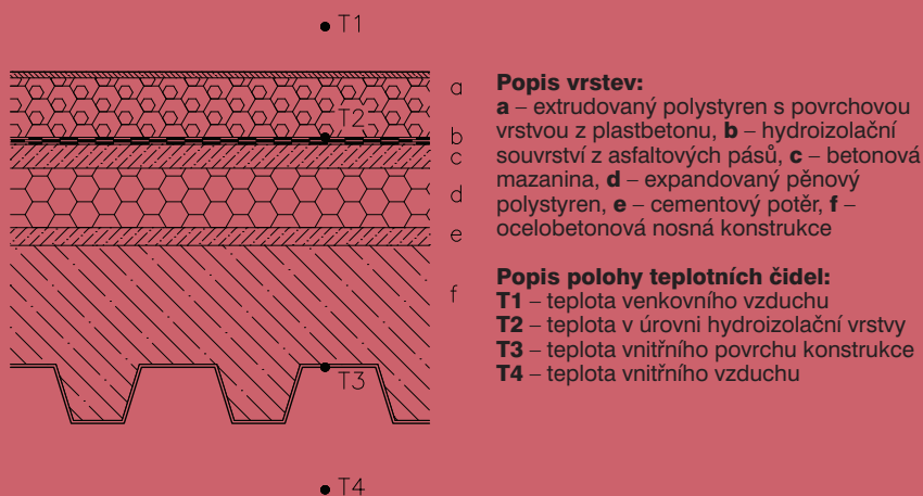
Obr. 01 | Schéma skladby pozorované střechy
