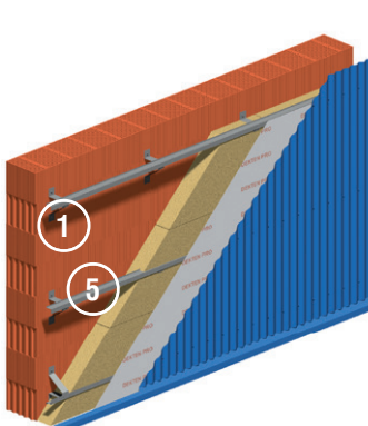
DKM1B Jednosměrný rošt vodorovný
