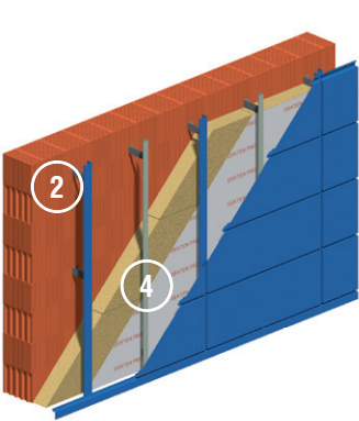
DKM1A Jednosměrný rošt svislý
