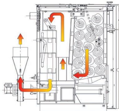
Schéma spalování
