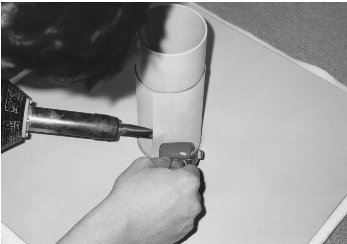
Obrázek 17.: Opracování vstupu - navaření pásu na kruhový vstup
