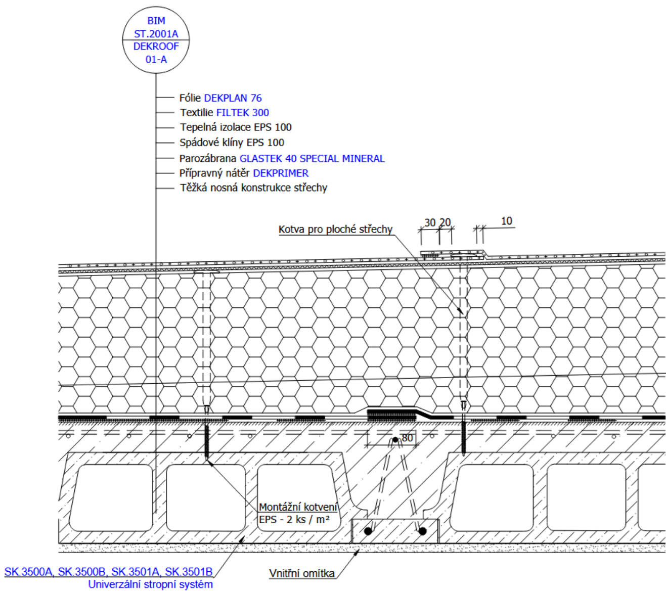
Detail 2.: Skladba jednovrstevné střechy, podélný spoj fólie s kotvením, geometrie spoje
