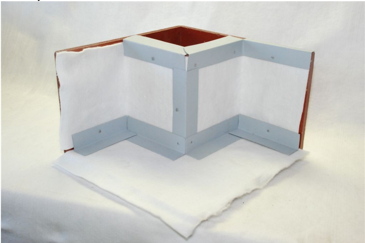
Obrázek 8.: Postup opravování hydroizolace v koutu - příprava hydroizolace
