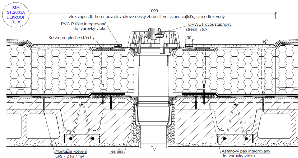
Detail 9.: Opracování střešního vtoku (manžetu vtoku je možné napojit na hydroizolaci z plochy jak ze spodní tak i z horní strany)
