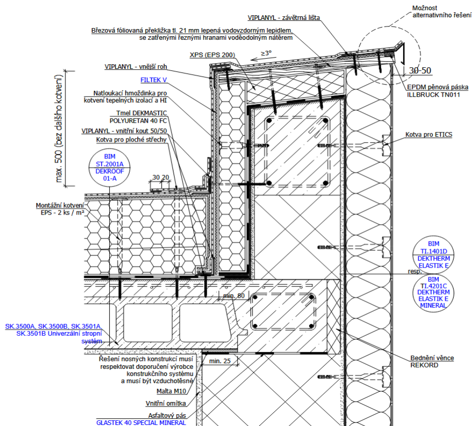
Detail 5.6.: Varianty ukončení hydroizolace na atice. U spodní varianty je možné v případě zkušeného izolátora vypustit vnitřní koutovou lištu.
