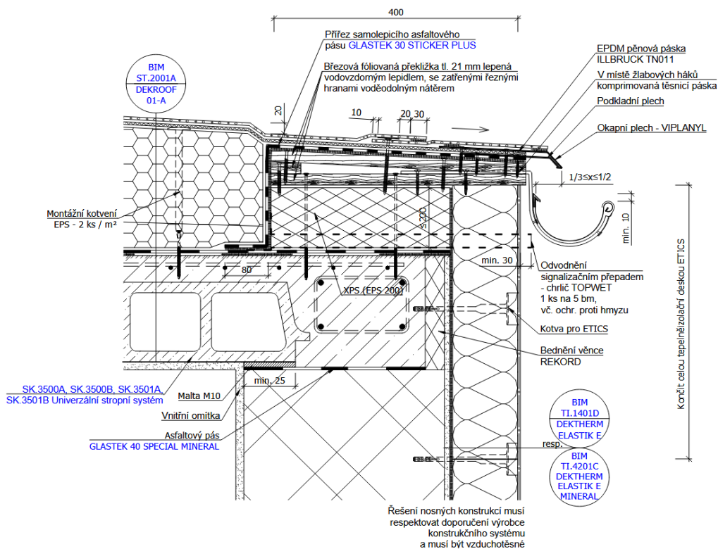
Detail 4.: Ukončení fólie na okapnici
