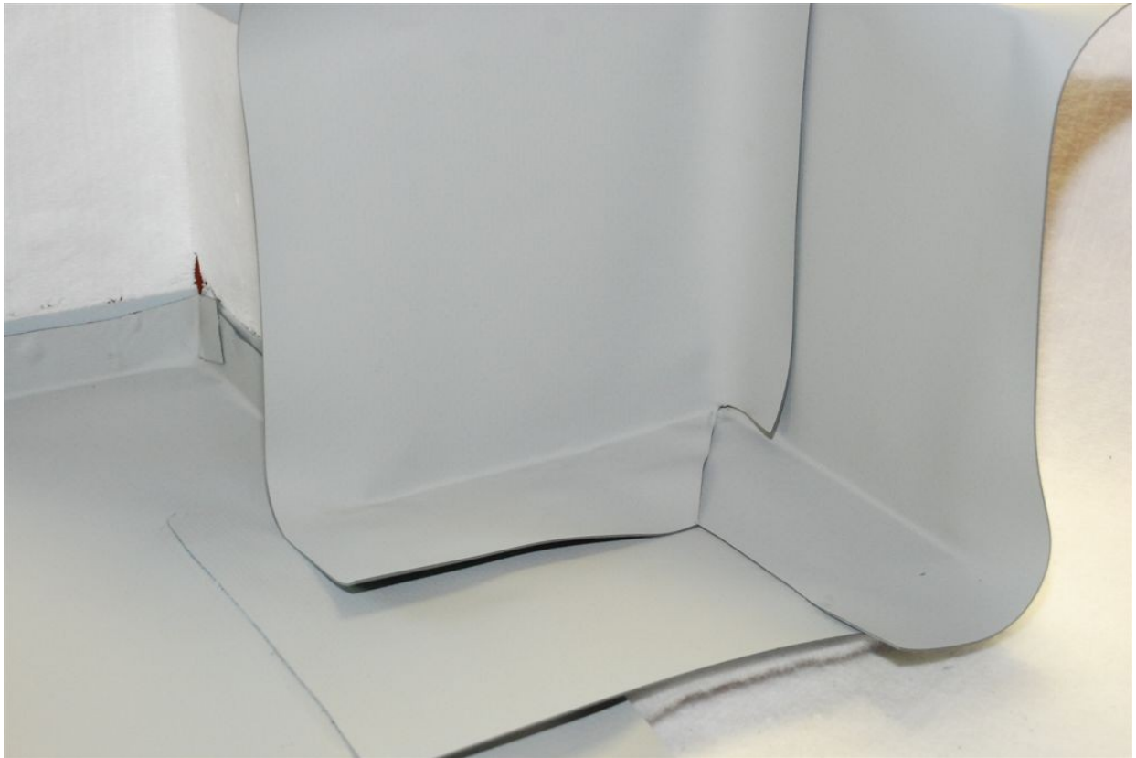
Obrázek 11.: Postup opravování hydroizolace v koutu
