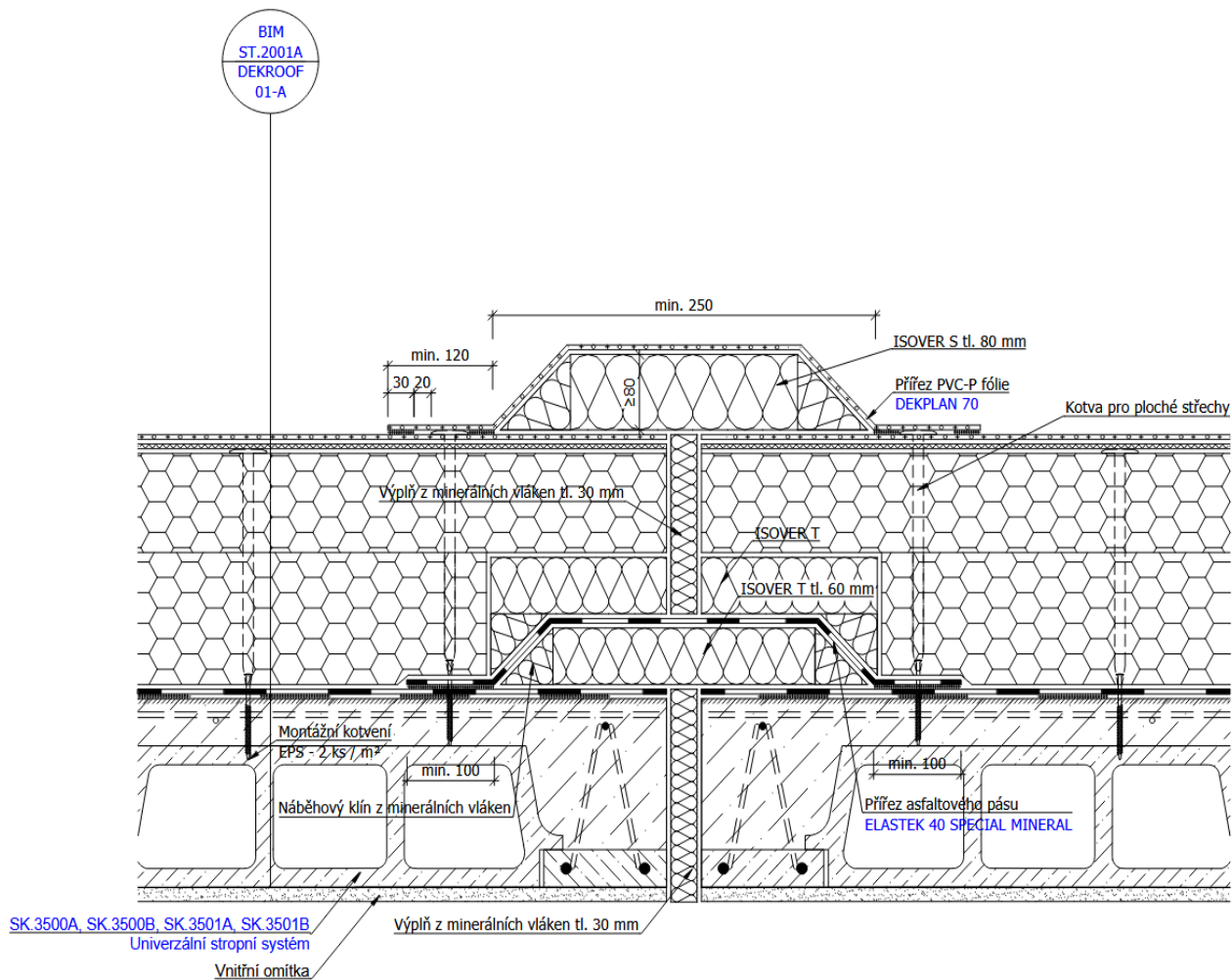
Detail 7.: Objektová dilatační spára svislý/vodorovný posun 20-30 mm
