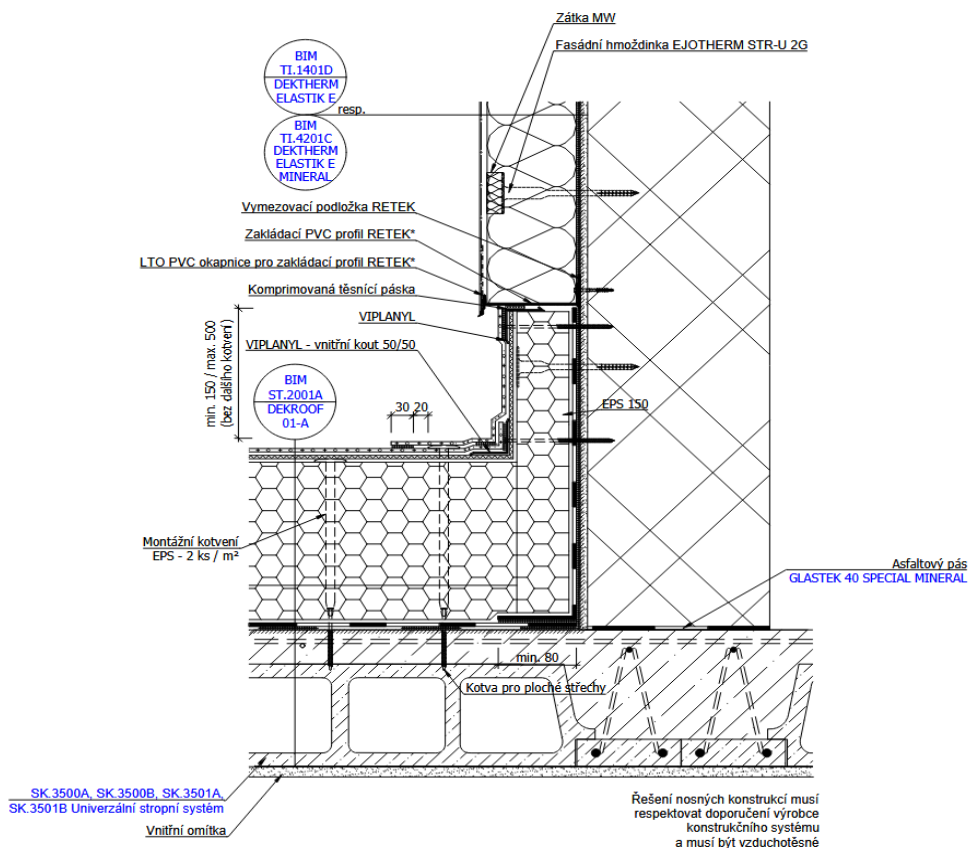
Detail 3.:Detail napojení vodorovné a svislé plochy, detail ukončení fólie na svislé ploše
