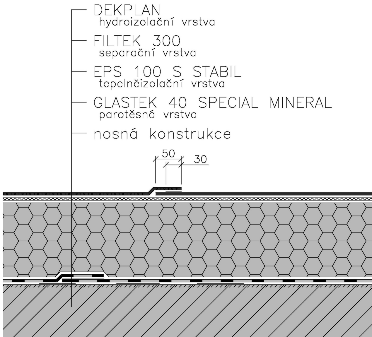
Detail 1.:Skladba jednovrstevné střechy, příčný spoj fólie bez kotvení, geometrie spoje
