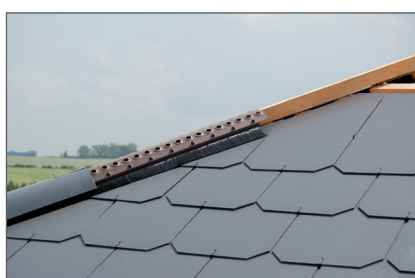
Velikost výstupního otvoru při větrání hřebenem je 100 cm 2 /bm. Větrací mezera 1 cm/bm.
