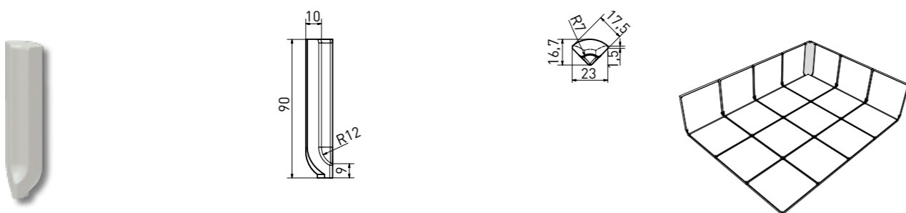
vnitřní roh sokl s požlábkem | inside corner cove skirting | TSIRB... | 90×23×10 mm*
