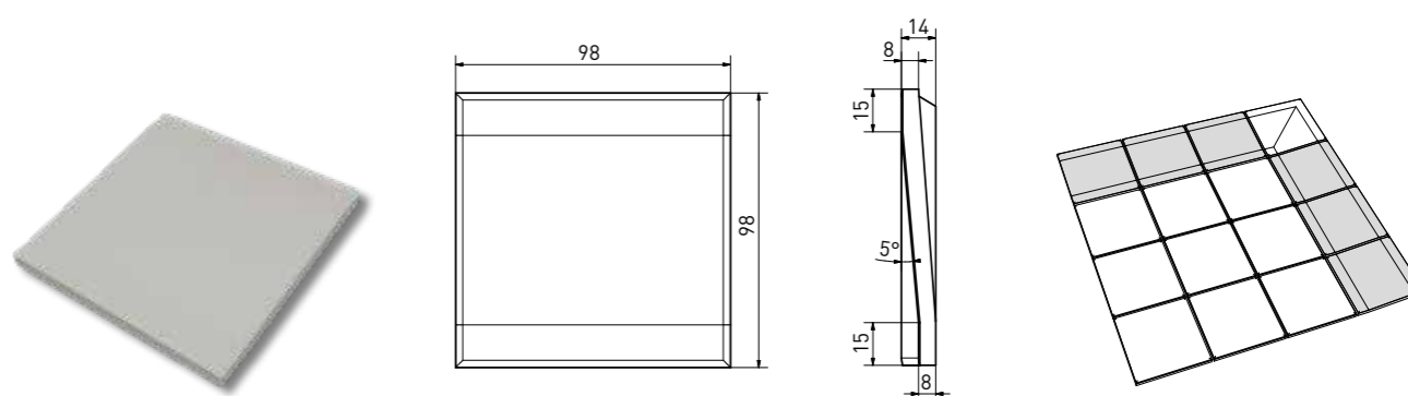
bezbariérová tvarovka průběžná | shower piece - continuous | TTP12... | 98×98×8 mm*
