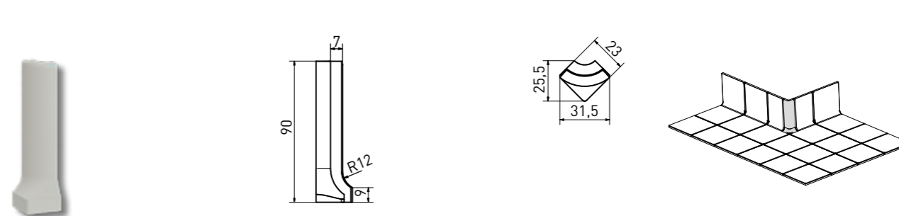
vnější roh sokl s požlábkem | outside corner cove skirting | TSERB... | 90×23×7 mm*
