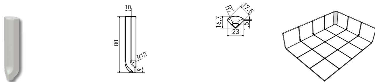
vnitřní roh sokl s požlábkem | inside corner cove skirting | TSIRH... | 80×23×10 mm
