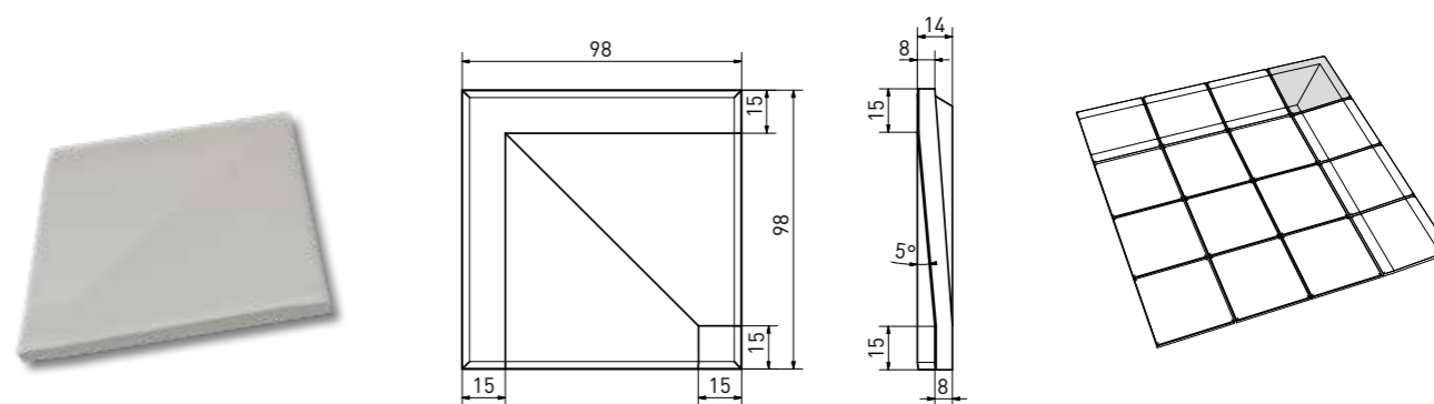
bezbariérová tvarovka rohová | shower piece - corner | TTR12... | 98×98×8 mm*
