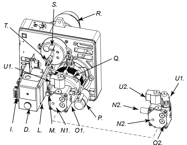
Figur 6 - Brennerens komponenter
