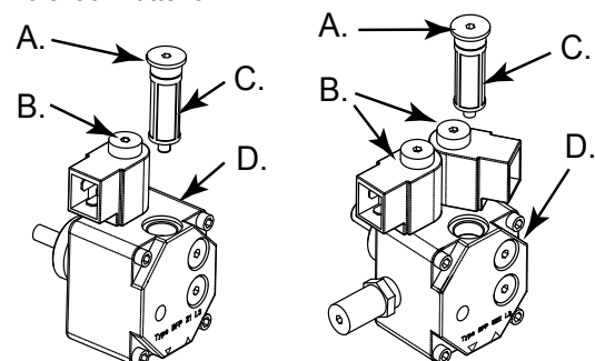
Kuva 11 - Polttimen pumppu
