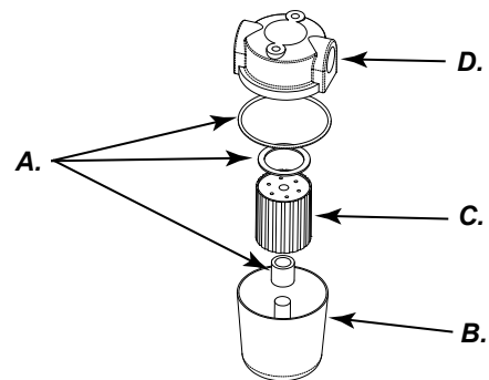
Kuva 10 - Suodatin
