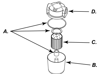
Рисунок 10 - Фильтр нагревателя
