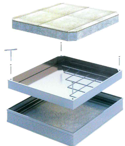
Ukázka poklopu DC-80 Pro-Line
