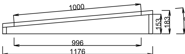
Pohled spodní
