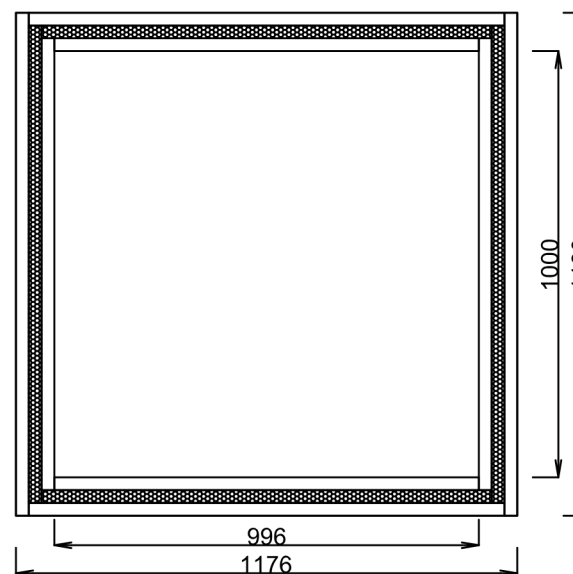
Pohled spodní
