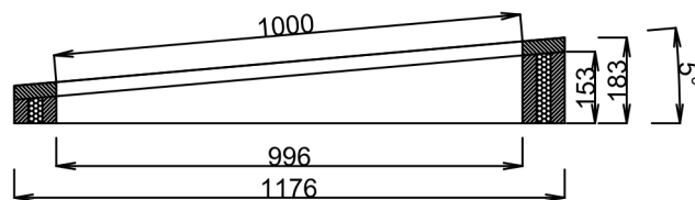
Základní profil
