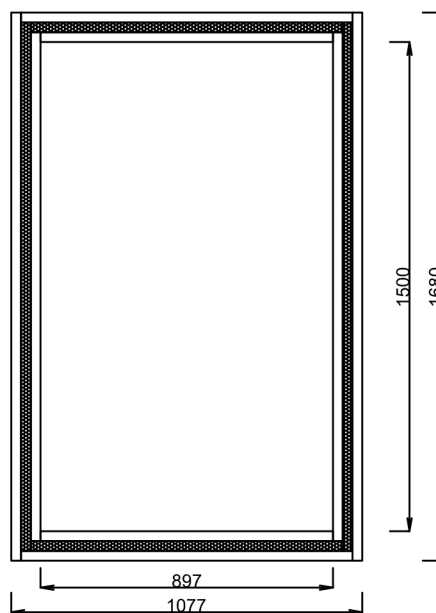
Pohled spodní
