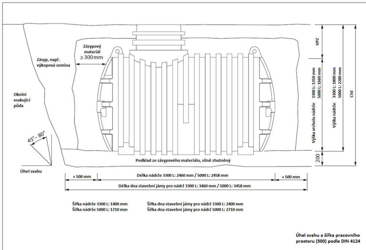
Obr. 2: Montážní velikosti
