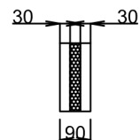
Základní profil
