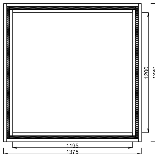
Pohled spodní
