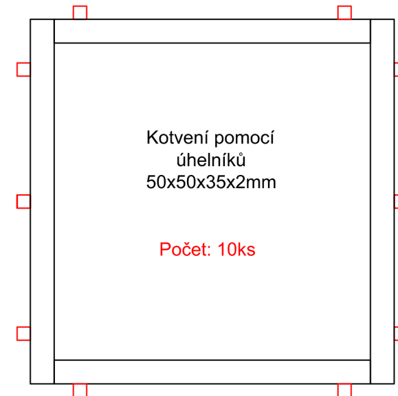
Pohled zadní
