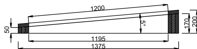
Řez příčný
