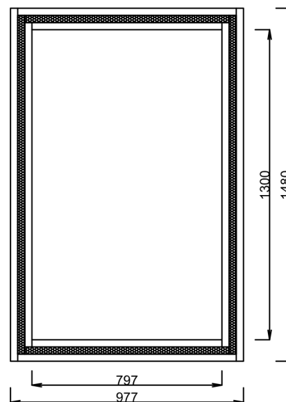
Pohled spodní
