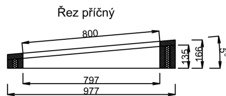
Základní profil
