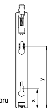
Rozmístění montážních otvorů pro T21,22,33
