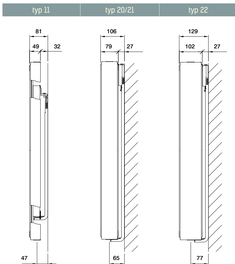
Rozmístění montážních otvorů Typ 11/20-22
