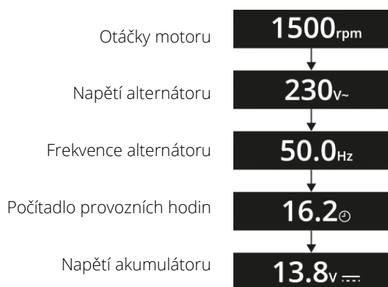
Obrázek 11: Parametry měřené ovládacím panelem DSE 3110
