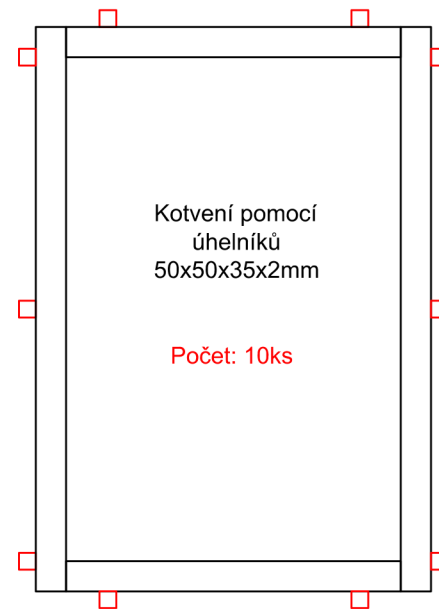
Pohled zadní
