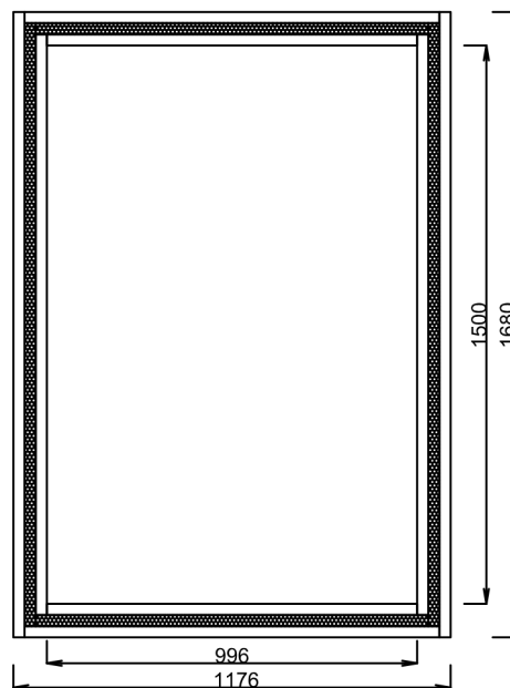
Pohled spodní
