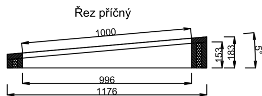
Základní profil
