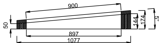
Řez příčný
