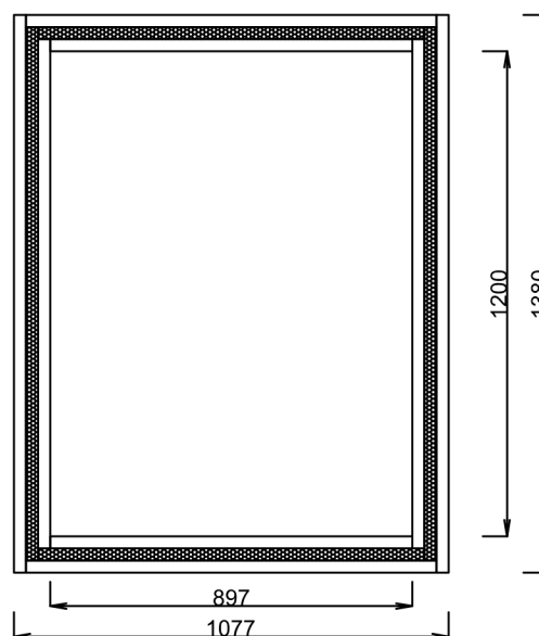
Pohled spodní
