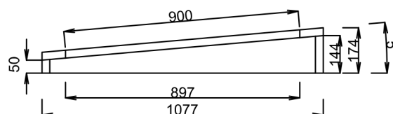
Pohled spodní
