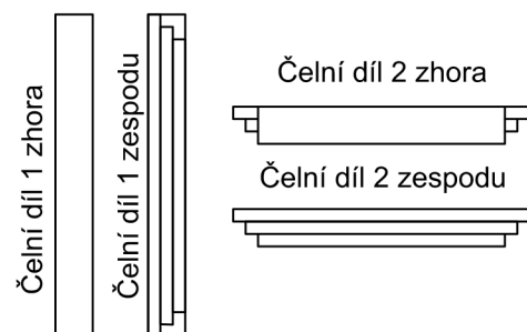
Jednotlivé díly rámu
