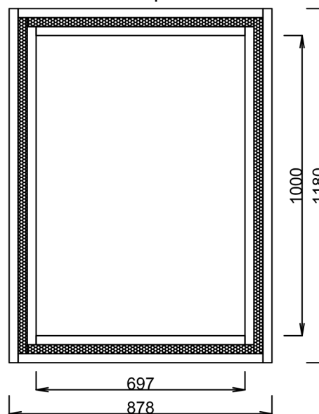
Pohled spodní
