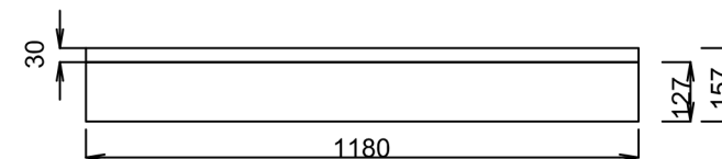
Pohled zadní
