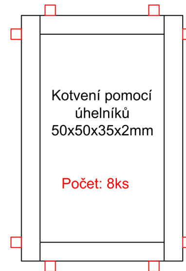
Pohled zadní
