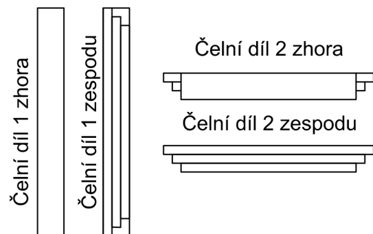
Jednotlivé díly rámu
