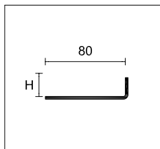
CPLB/2 základna s drenážními otvory pro keramické dlažby
