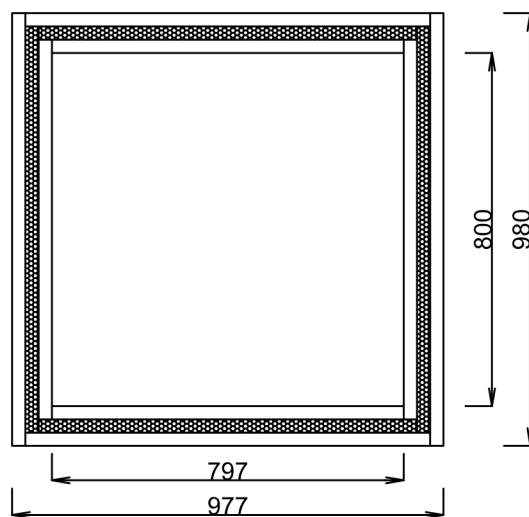
Pohled spodní
