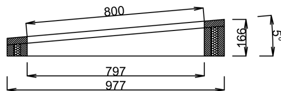
Základní profil
