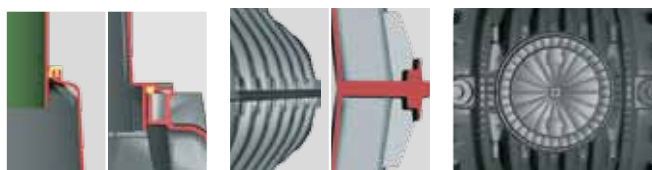
1. Utěsněno až po horní hranu terénu (2 těsnění)
