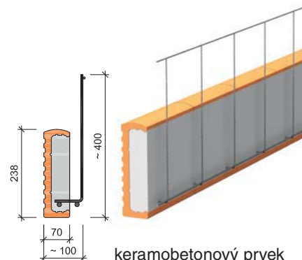
keramobetonový prvek KP Vario 200 až 350
