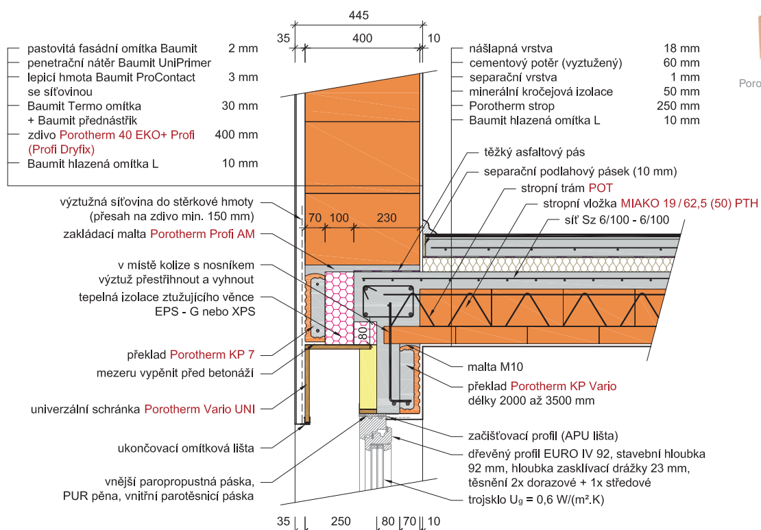
Příklad Porotherm KP Vario UNI délky 2 000 až 3 500 mm ve stěně tl. 400 mm, strop tl. 250 mm
