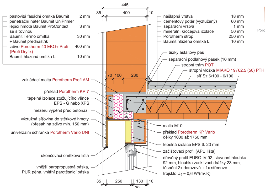
Příklad Porotherm KP Vario UNI délky 1 000 až 1 750 mm ve stěně tl. 400 mm, strop tl. 250 mm
