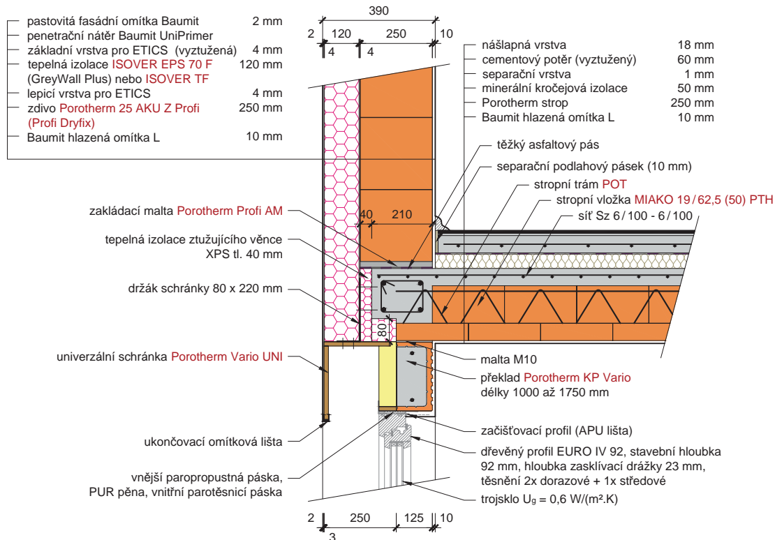
Překlad Porotherm KP Vario UNI délky 1 000 až 1 750 mm ve stěně tl. 250 mm + ETICS, strop tl. 250 mm
