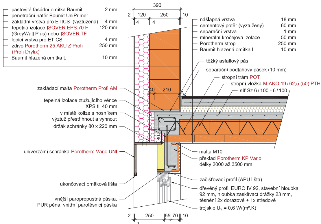
Překlad Porotherm KP Vario délky 2 000 až 3 500 mm ve stěně tl. 250 mm + ETICS, strop tl. 250 mm
