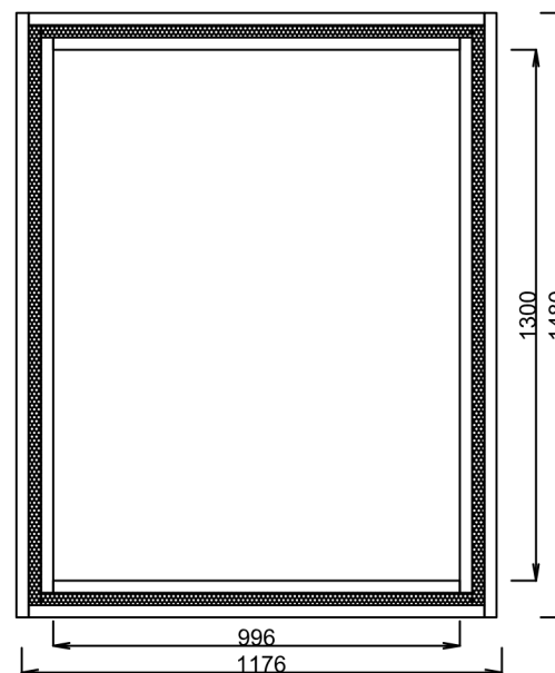
Pohled spodní
