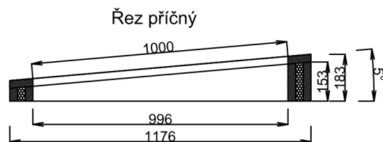
Základní profil
