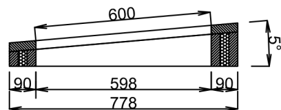
Základní profil
