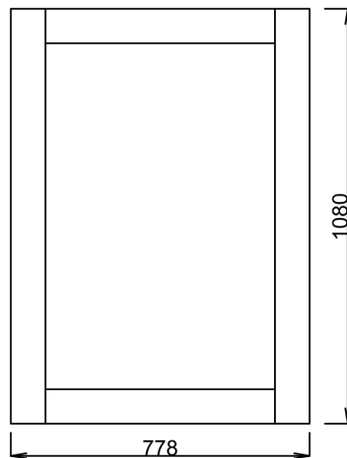
Pohled zhora
