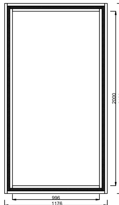
Pohled spodní
