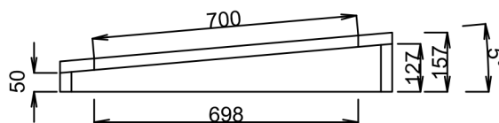
Pohled boční
