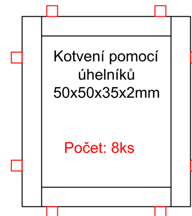
Pohled zadní
