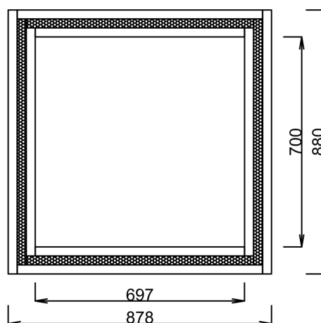
Pohled spodní
