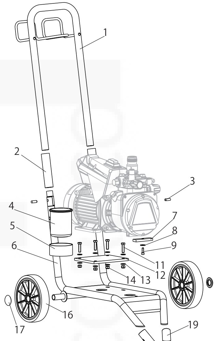
Diagram náhr. dílů vozík
