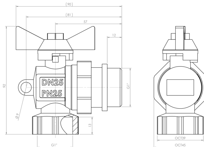
Rozměrová schéma rohového kulového kohoutu DEK SKR2
