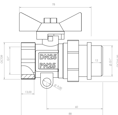
Rozměrová schéma přímého kulového kohoutu DEK SKR1
