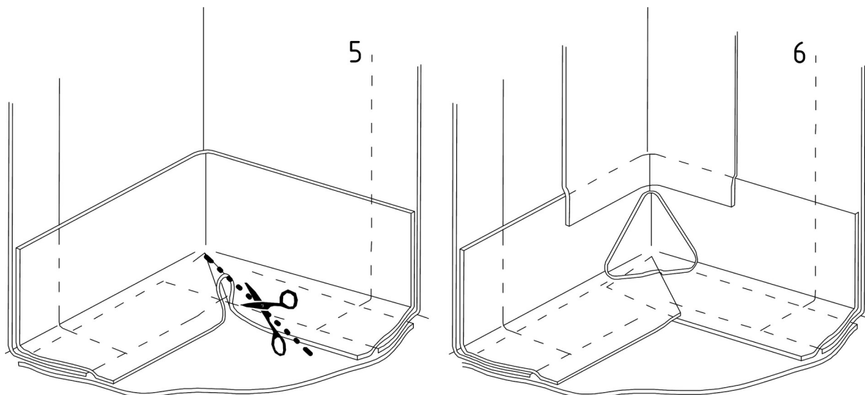
Schéma 8b - Provádění jednovrstvé izolace v koutu – vyztužení koutů
