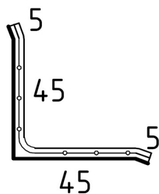
Schéma 1 - Typizované spojovací profily z plechu s vrstvou PVC-P
