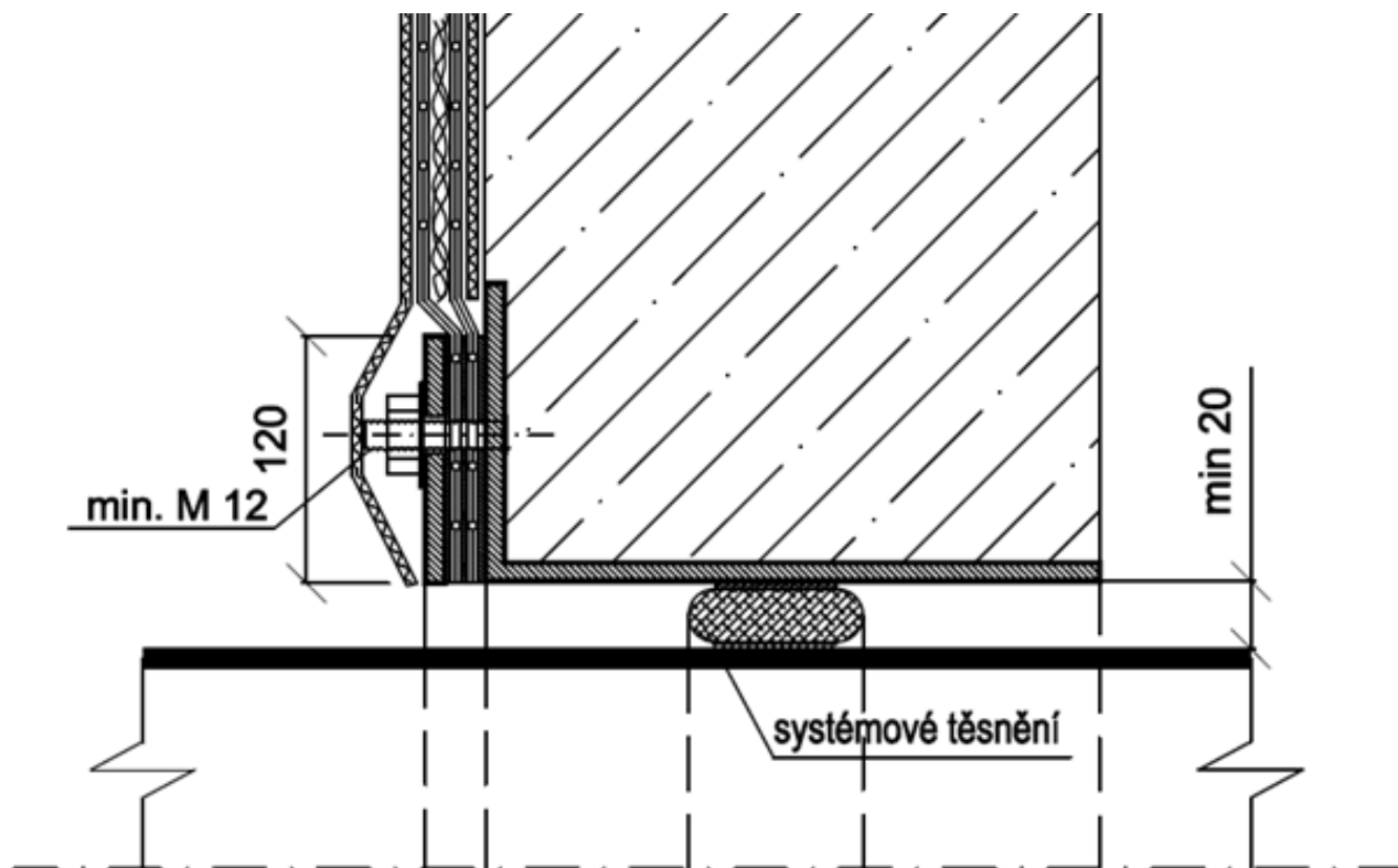
Schéma 17 - Prostup izolací v podmínkách tlakové vody, příklad utěsnění prostupu
