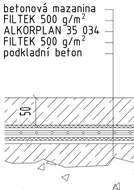
Schéma 6 - Ochrana vodorovné hydroizolace
