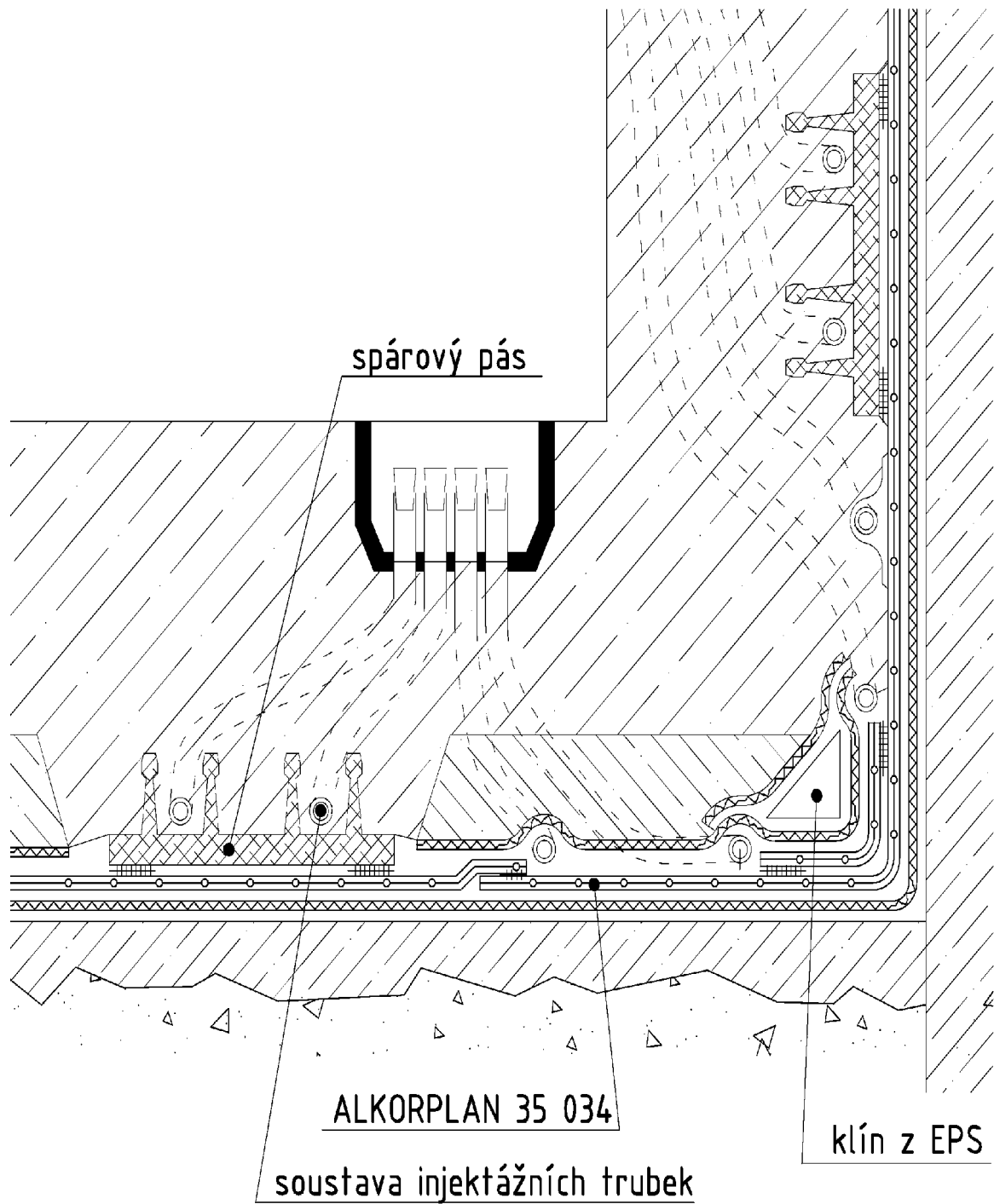
Schéma 2 - Princip jednovrstvého systému s možností sanace
