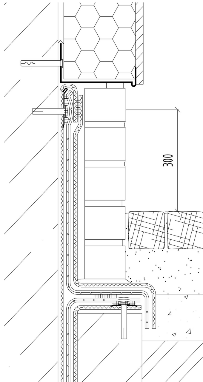
Schéma 11 - Příklad ukončení hydroizolace nad terénem s ochrannou přízdívkou a etapový spoj
