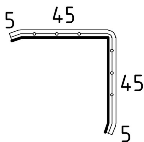
Schéma 1 - Typizované spojovací profily z plechu s vrstvou PVC-P
