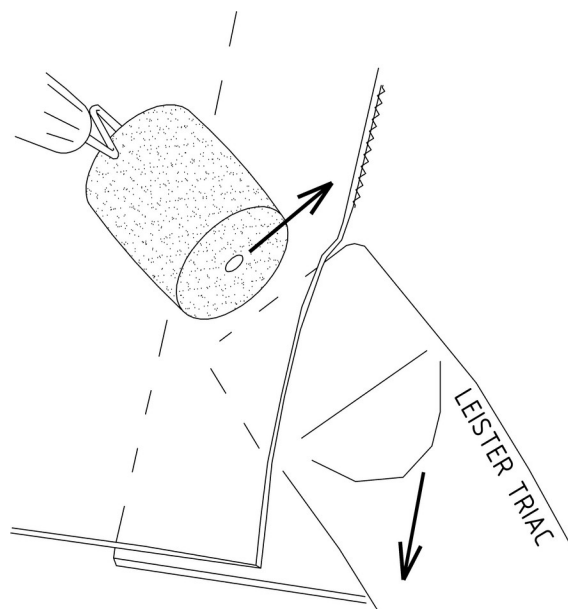
Schéma 4 - Práce s horkovzdušným přístrojem a válečkem
