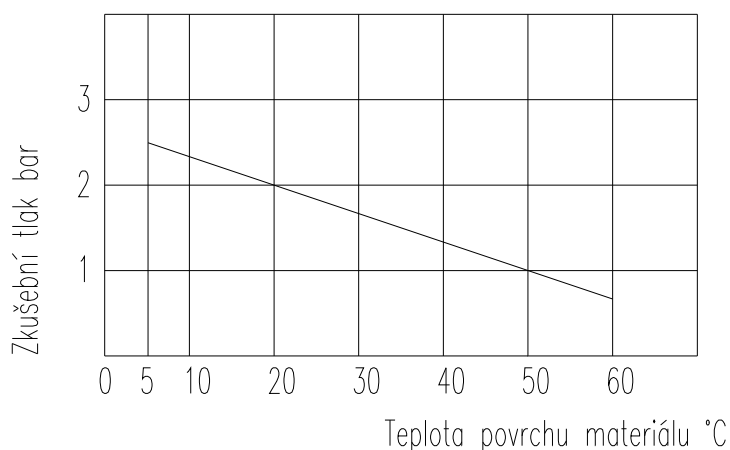
Schéma 19 - Graf závislosti zkušební tlaku na teplotě fólie při tlakové zkoušce
