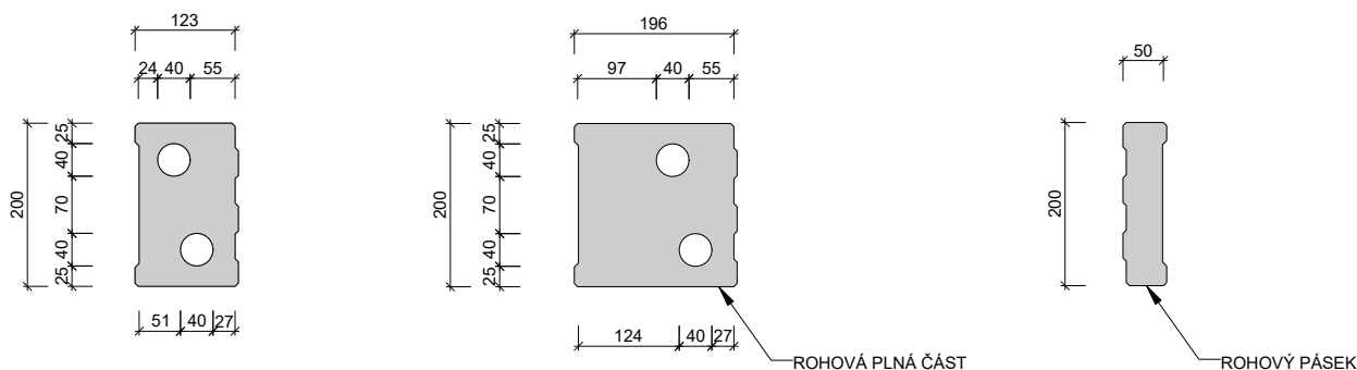
Broušená akustická betonová tvárnice BR 20 AKU
