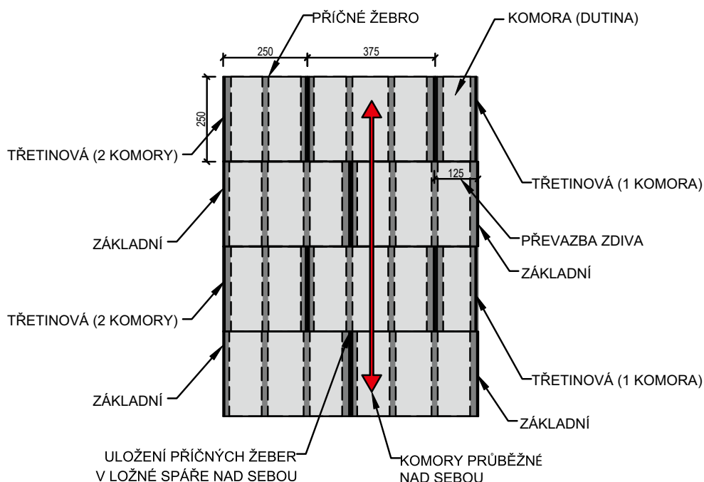
Broušené betonové tvárnice BR 25
