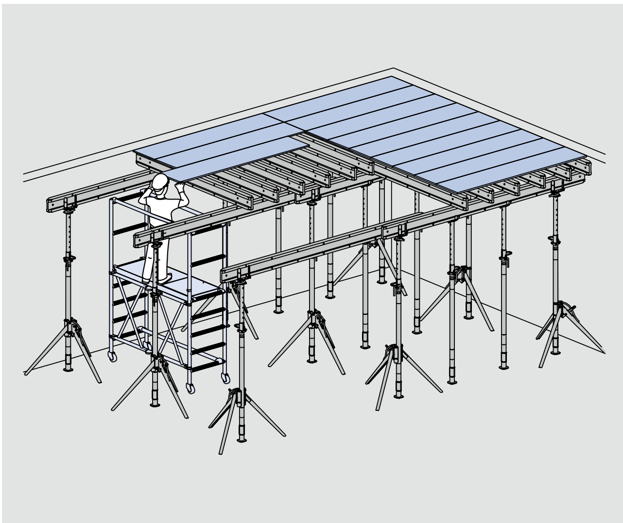
Obrázek 8 | Ukládání bednicích desek
