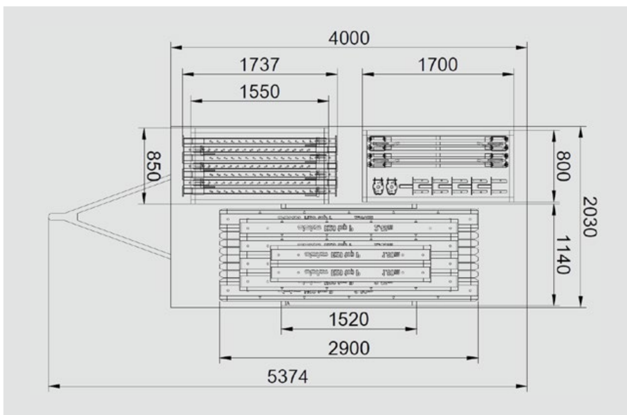
Příklad umístění přepravních prostředků Sestavy stropního bednění bez desek 45 m 2 na přívěs 4x2 m (PSK0459).
