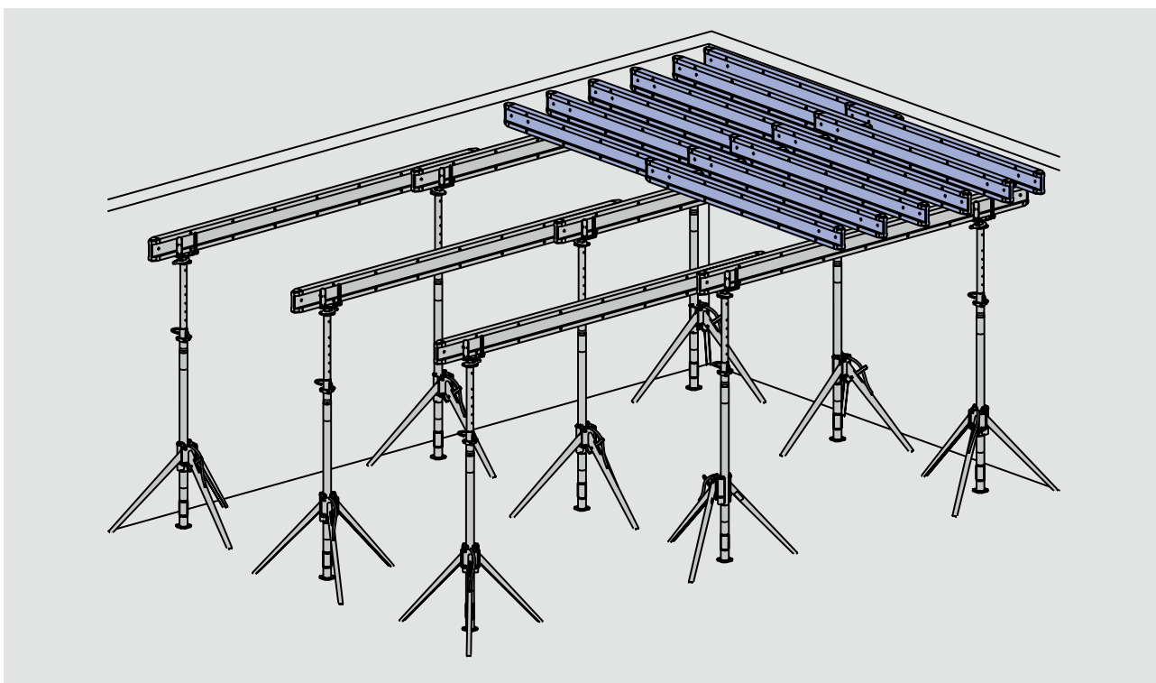
Obrázek 5 | Uložení příčných nosníků
