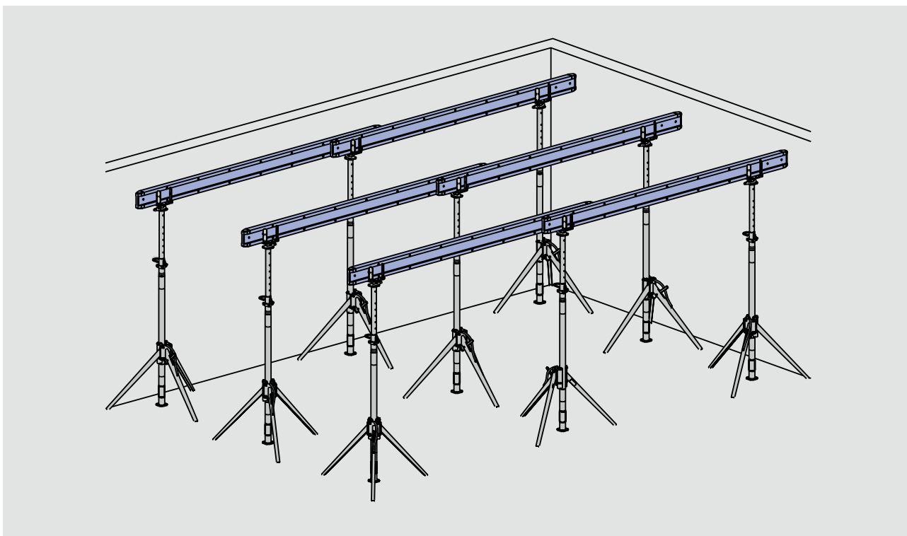
Obrázek 4 | Hotové podélné řady
