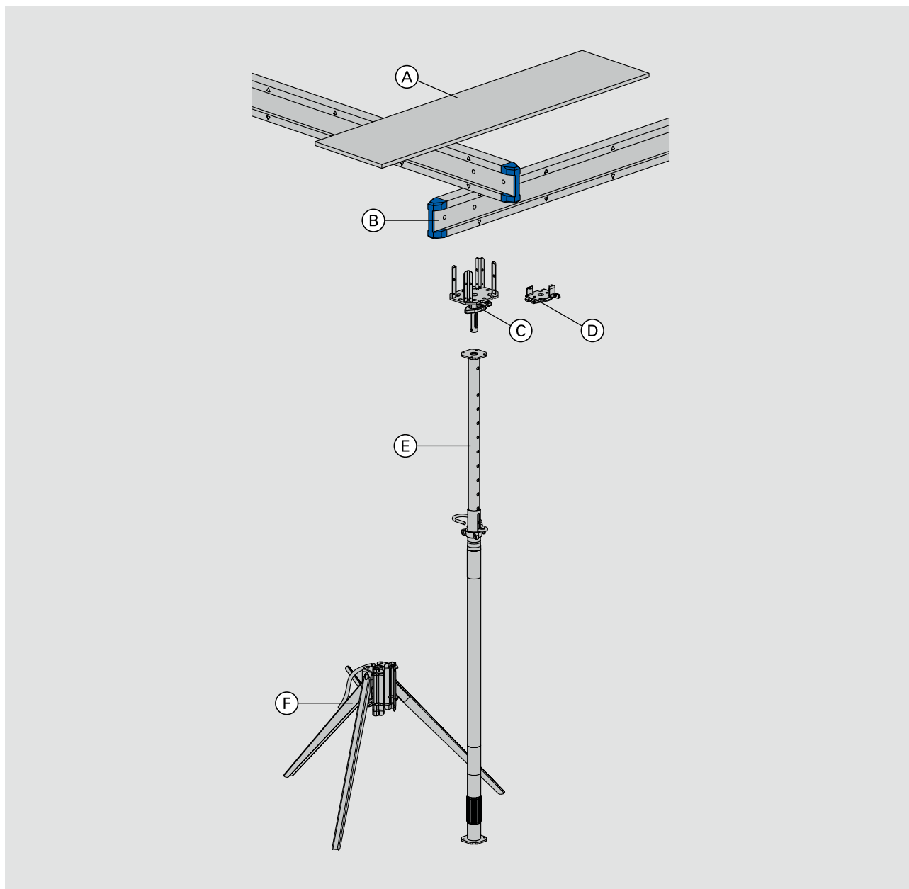
Obrázek 1 | Schéma komponent Dokaflex
