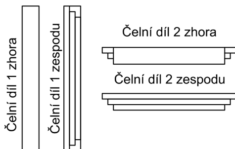
Jednotlivé díly rámu
