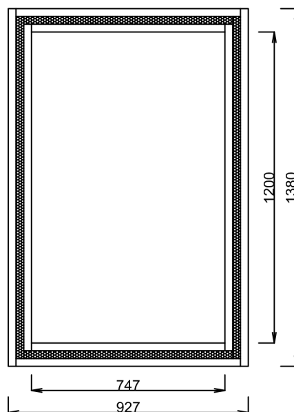
Pohled spodní
