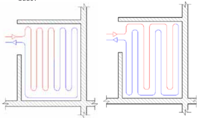
Jednoduchá serpentina
