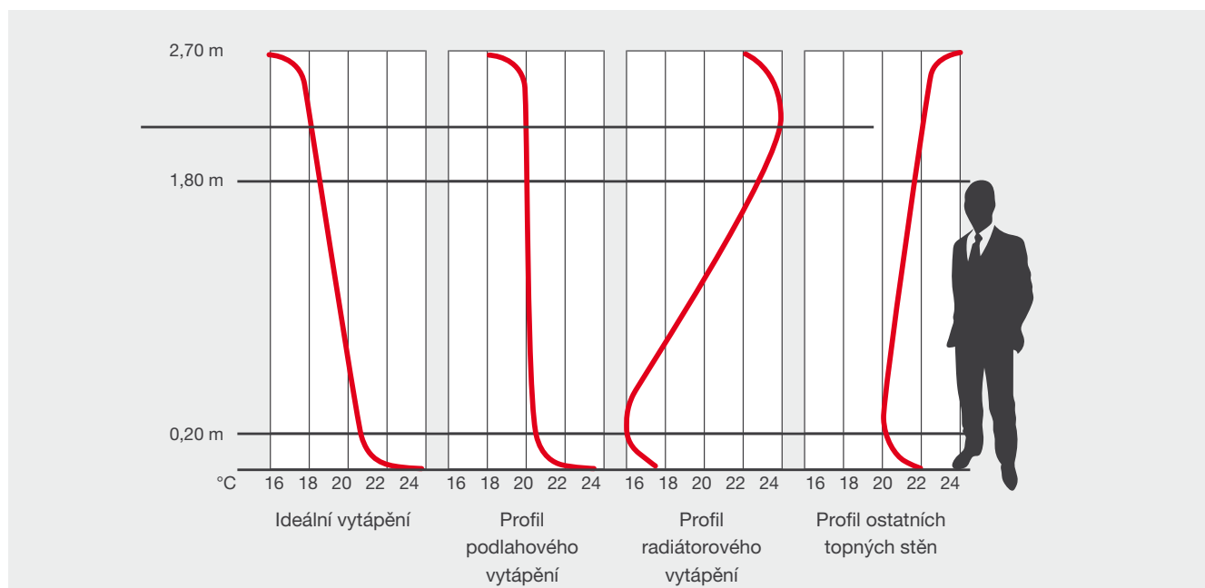
Tepelní profily různých systémů vytápění
