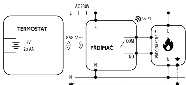
a) Schéma připojení k plynovému kotli
