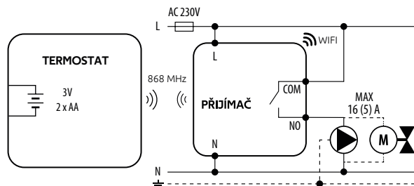
b) Schéma připojení k čerpadlu / pohonu ventilu
