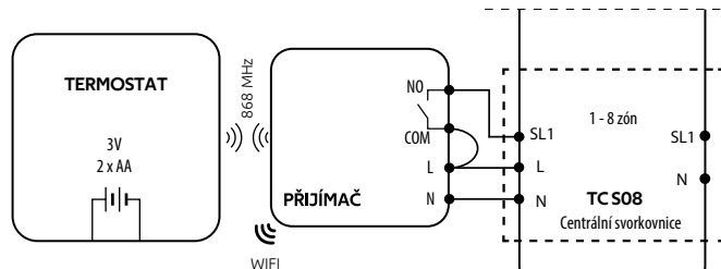
c) Schéma připojení k centrální svorkovnici
