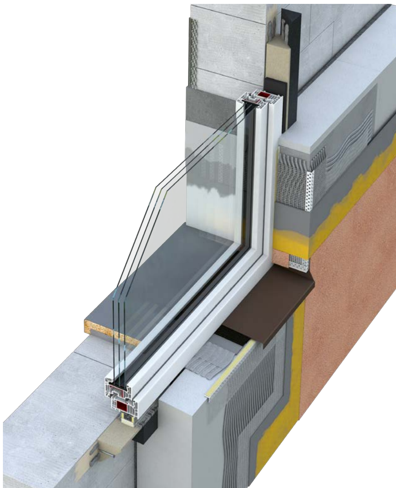
Předsazená montáž se systémem illbruck s vyložním 90 mm
