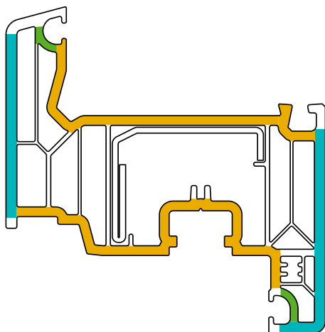
Profil křídla
