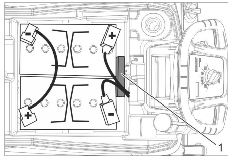
Batterie 6.654-141.0 1 Abstandshalter
