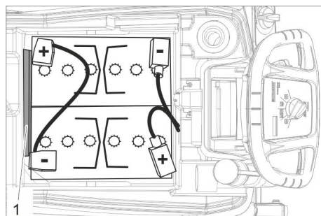
Baterai 6.654-290.0
