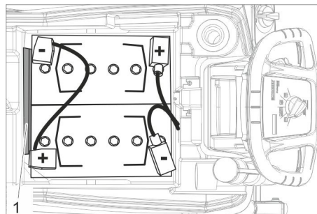
Batterie 6.654-093.0 1 Abstandshalter
