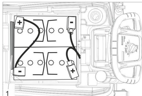
Batterie 6.654-290.0 1 Abstandshalter
