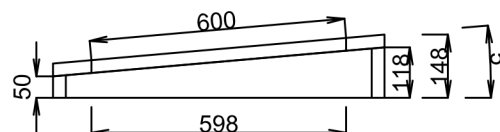
Pohled boční
