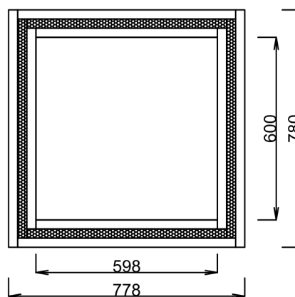
Pohled spodní
