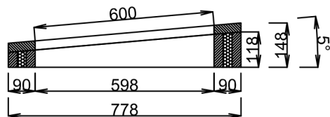
Základní profil
