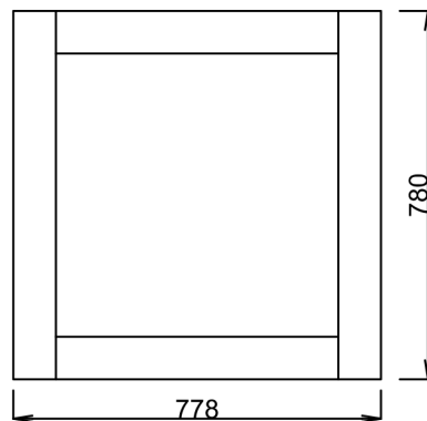
Pohled zhora
