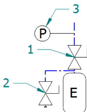
Obr 203 Zapojení expanzní nádoby
